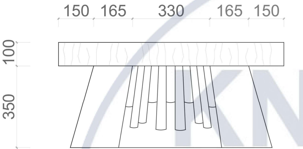
ВИД СПЕРЕДУ М 1:10
