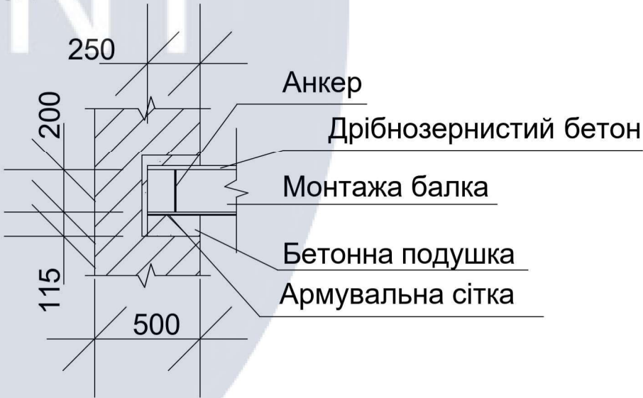
Вузол "А"
