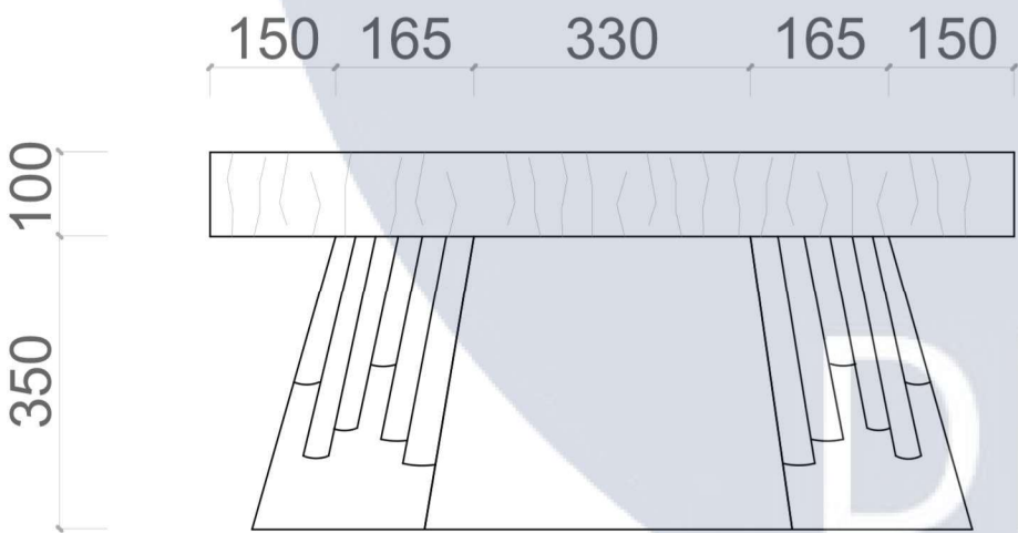
ВИД ЗБОКУ М 1:10
