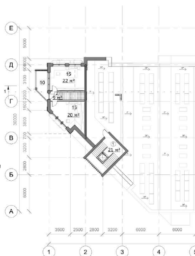
ПЛАН НА ВІДМІТЦІ +24.000
