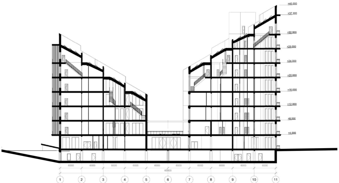
РОЗРІЗ 1-1
