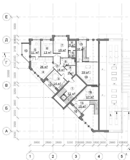
ПЛАН НА ВІДМІТЦІ +16.000
