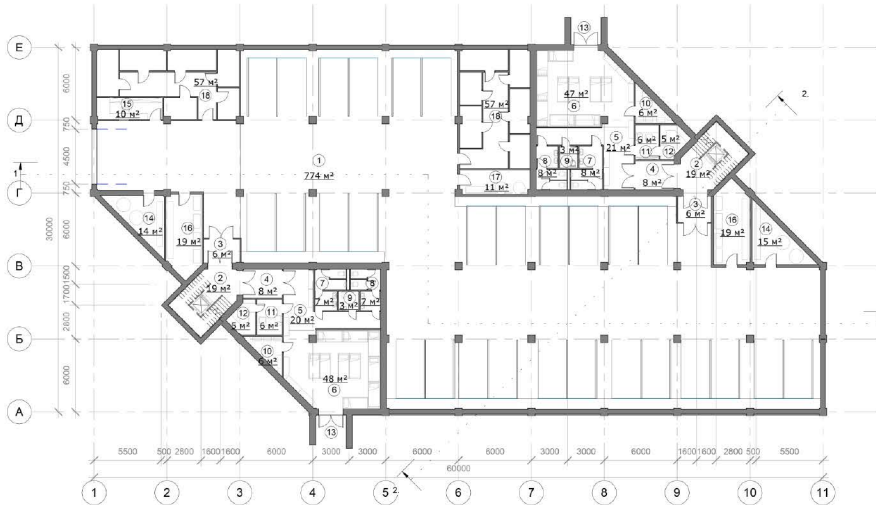
ПЛАН НА ВІДМІТЦІ -3.500
