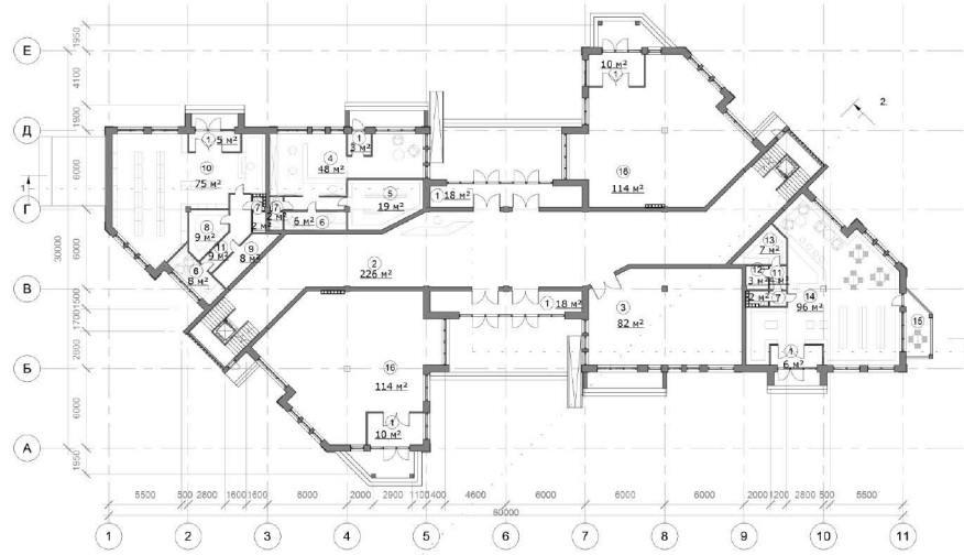
ПЛАН НА ВІДМІТЦІ +0.000
