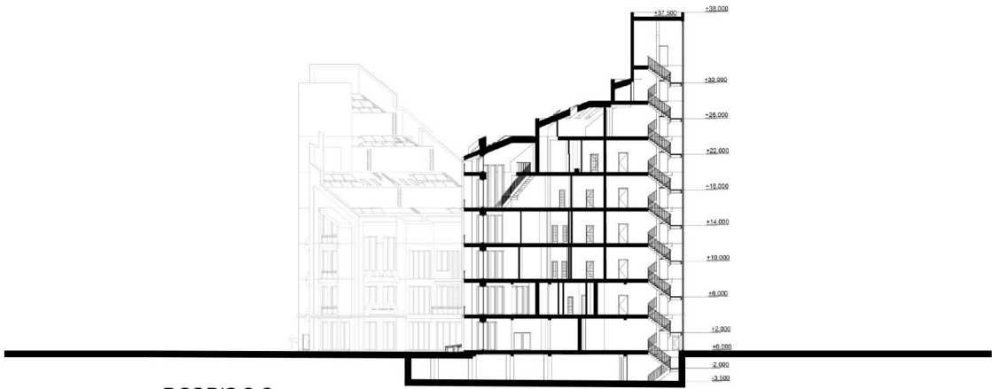
РОЗРІЗ 2-2
