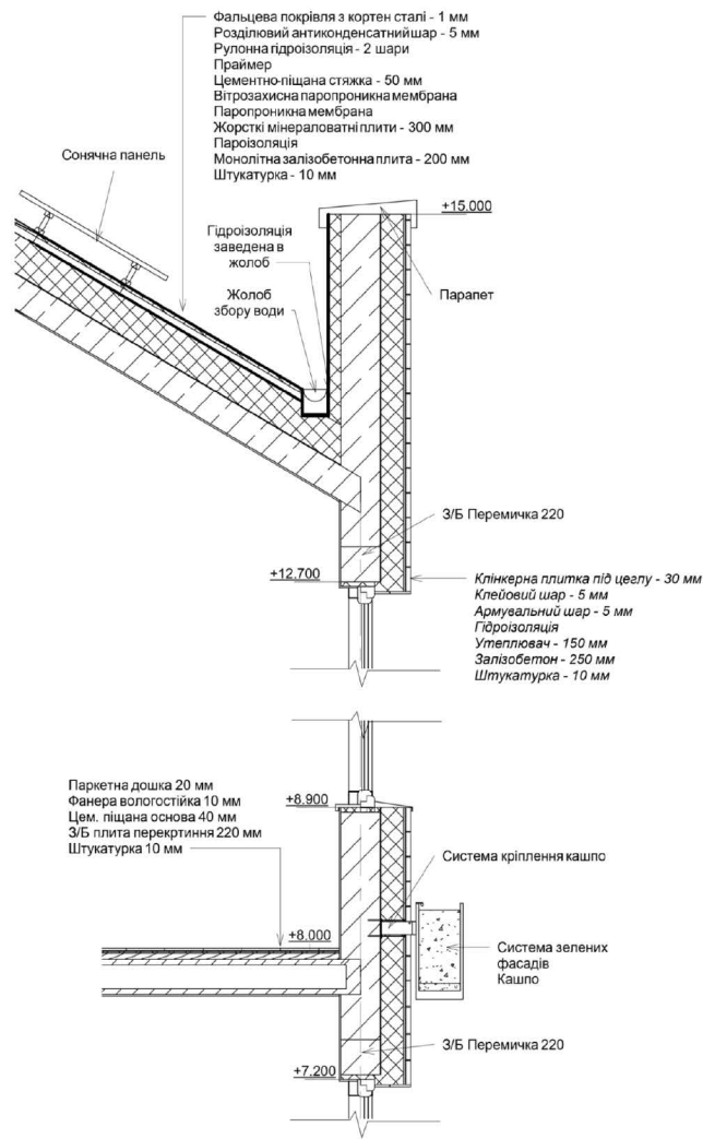
РОЗРІЗ 3-3
