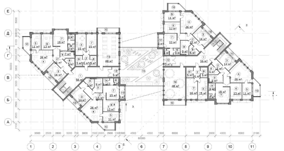
ПЛАН НА ВІДМІТЦІ +4.000
