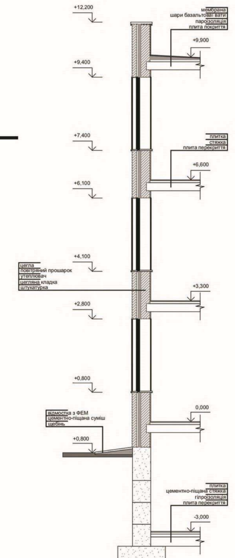
Конструктивний розріз по довільній стіні M1:25
