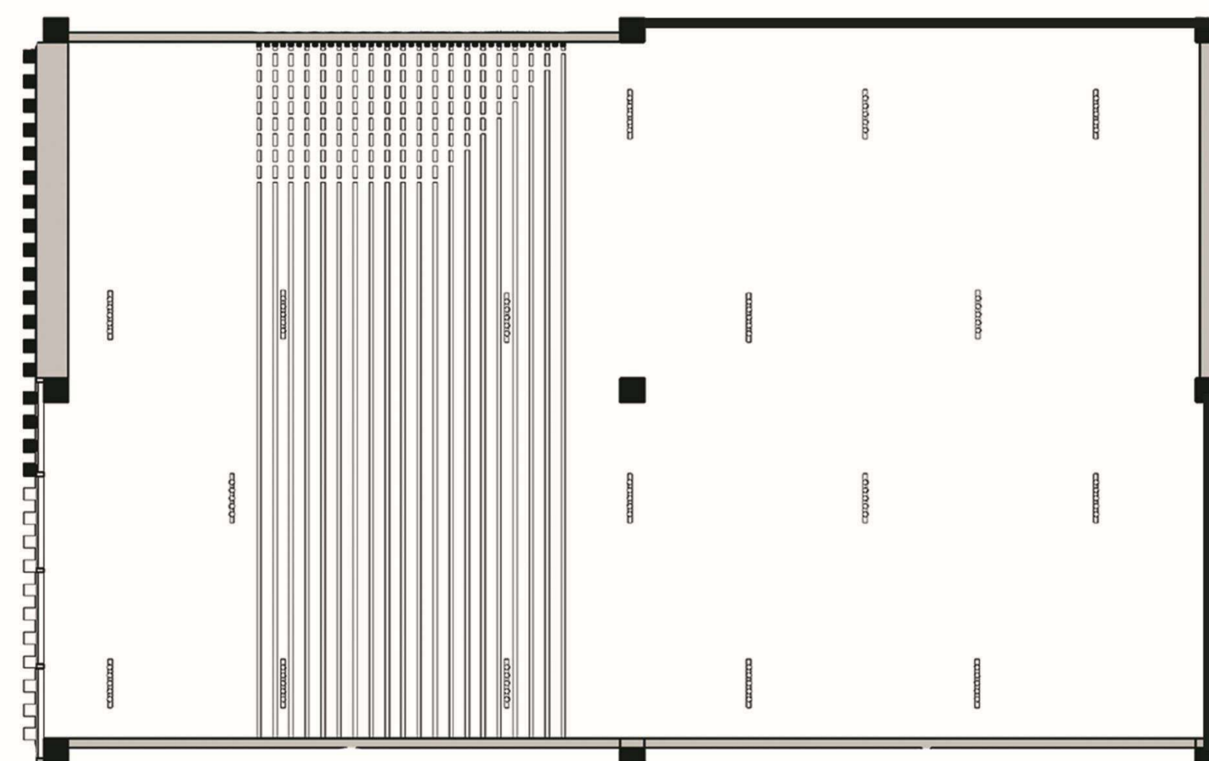
План стелі М1:50
