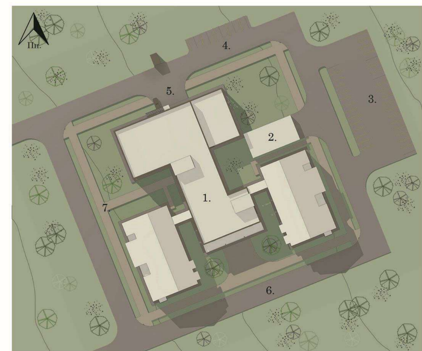
Генеральний план M1:500
