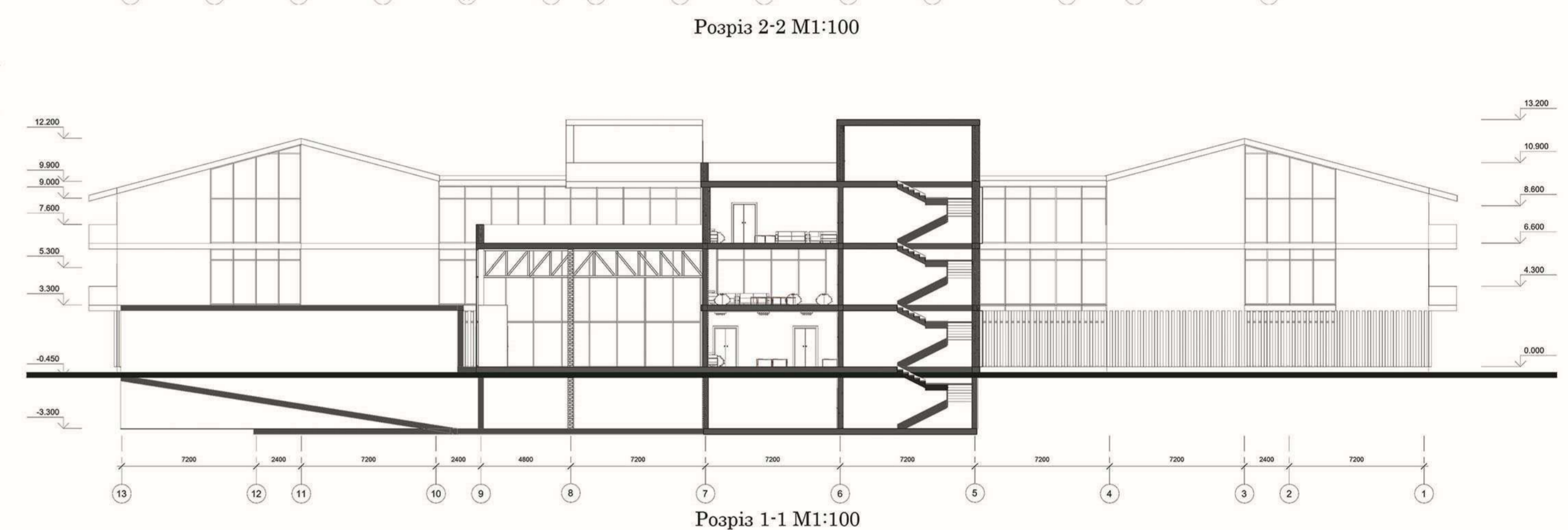
Розріз 1-1 M1:100
