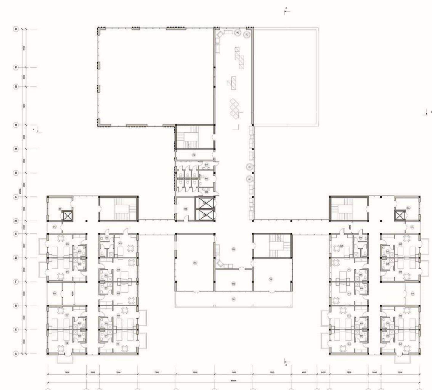
План на відс. +6.600 M1:200
