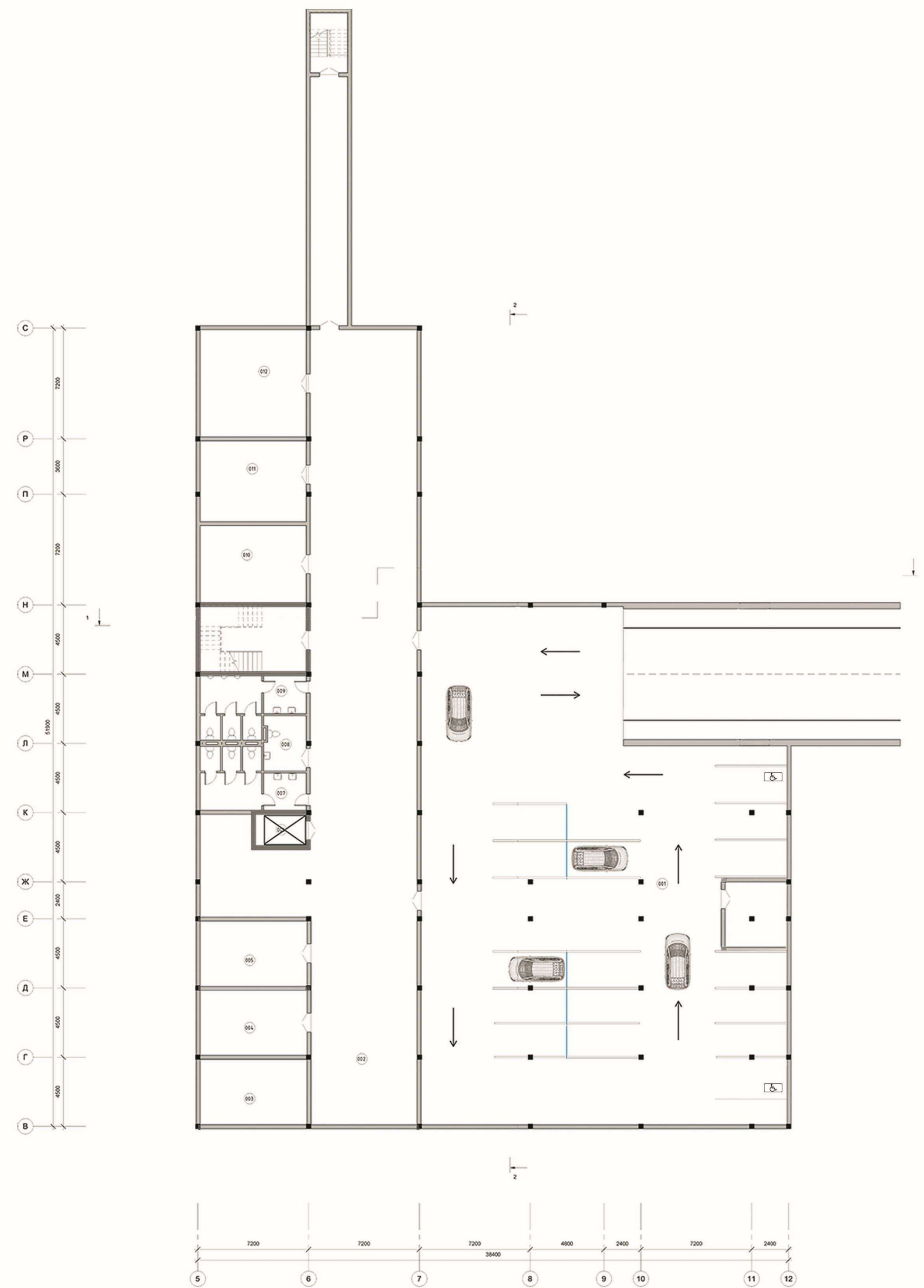
План на відм. -3.300 M1:100
