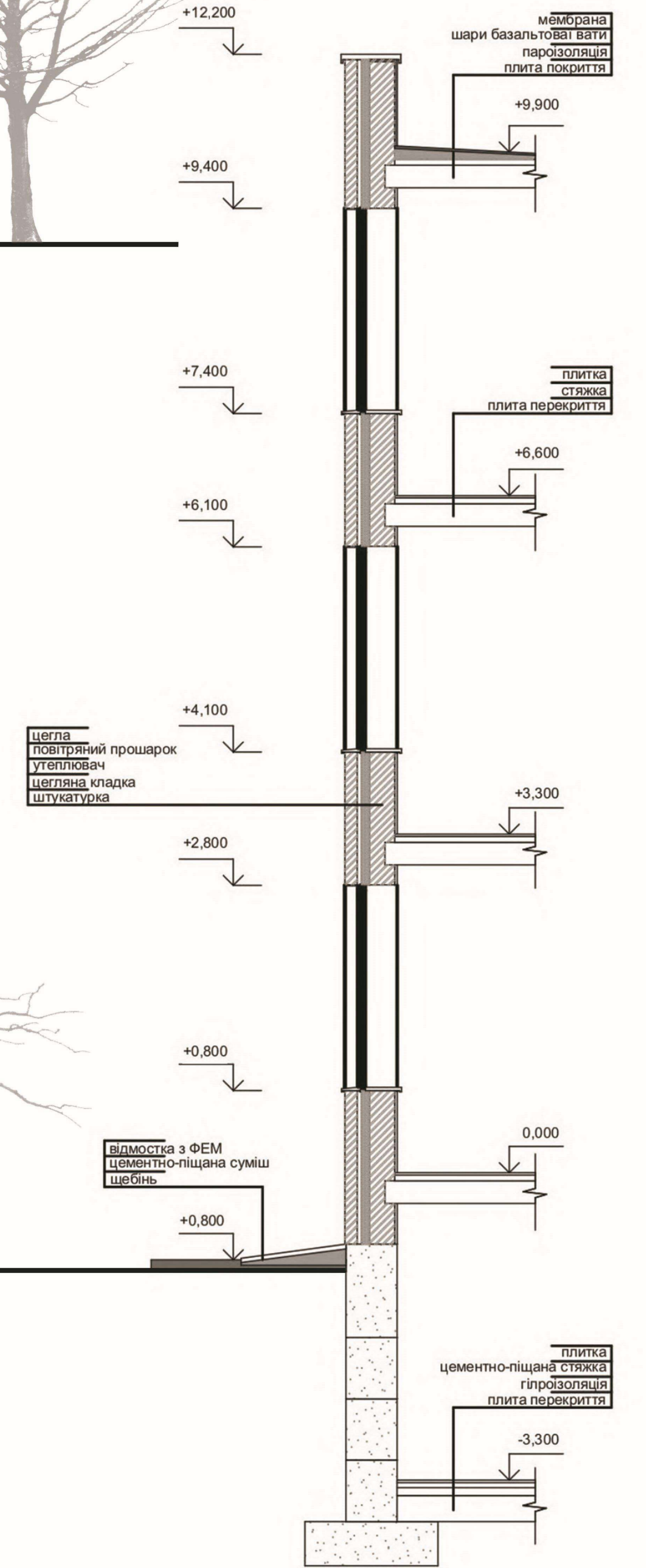
Конструктивний розріз по зовнішній стіні M1:25
