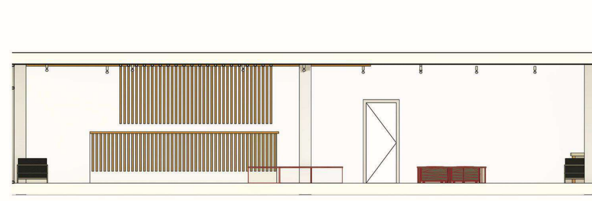
Розгортка по стіні 1-1 M1:50
