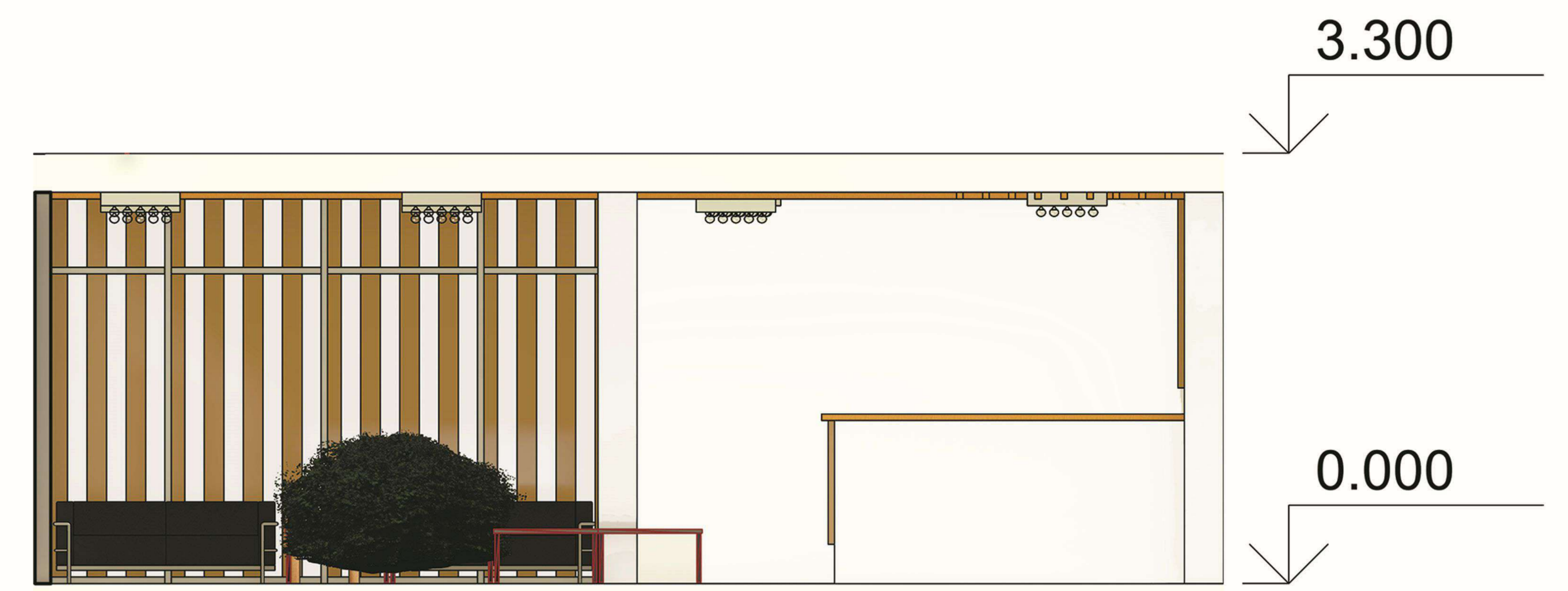
Розгортка по стіні 3-3 М1:50
