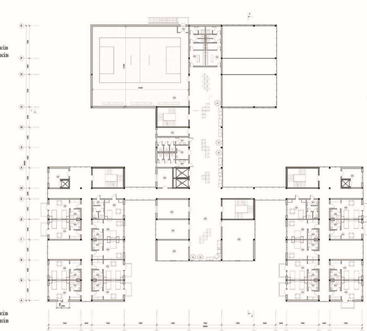
План на відс. +3.300 M1:200
