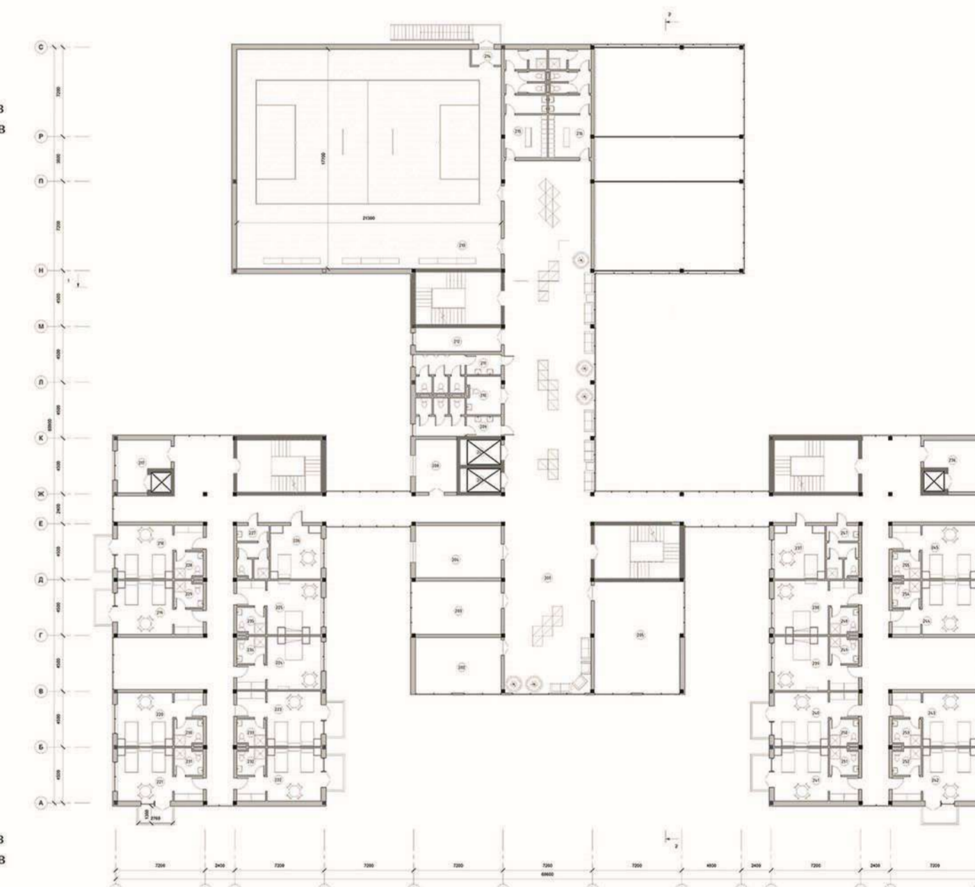
План на відм. +3.300 M1:200
