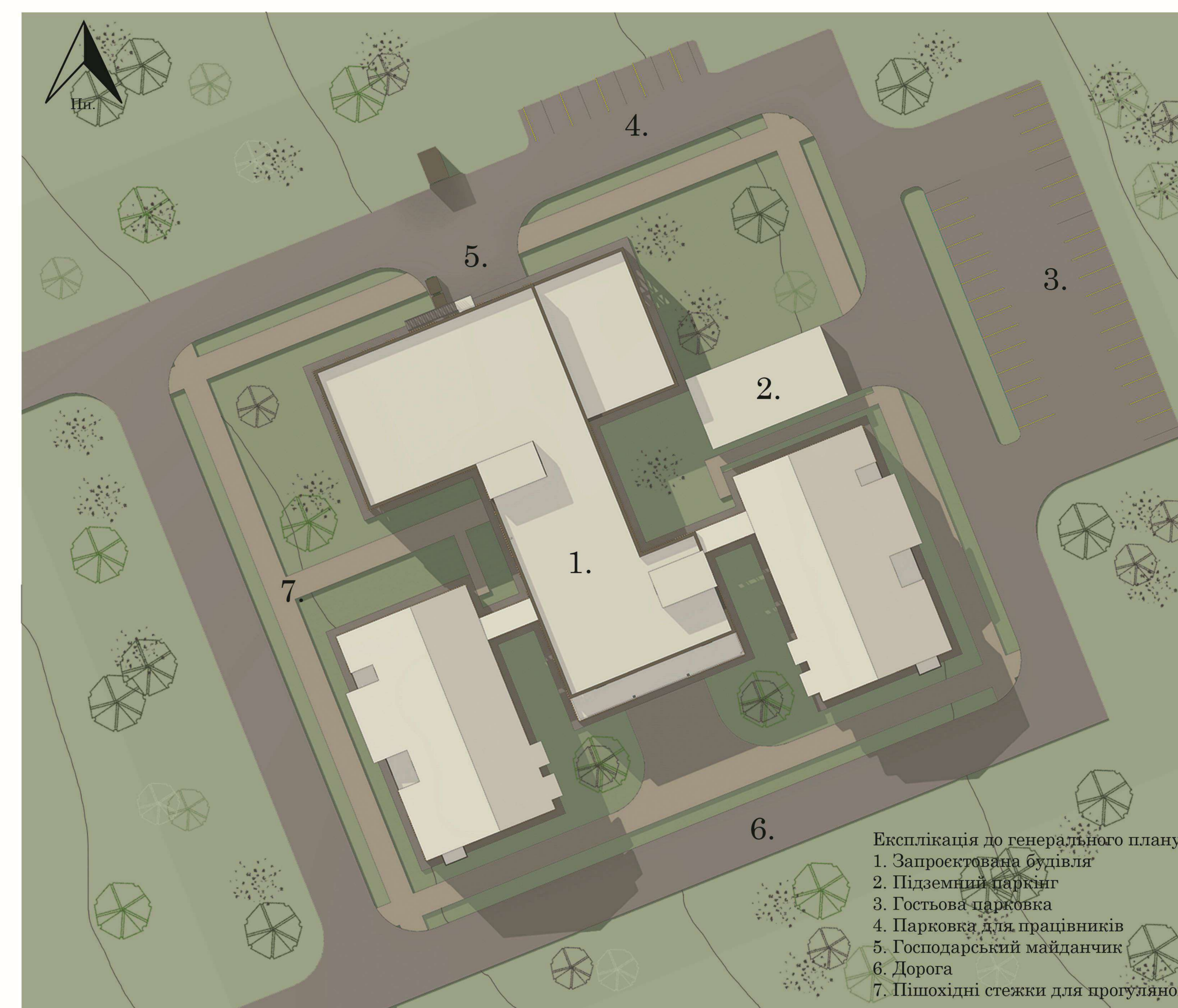
Генеральний план М1:500
