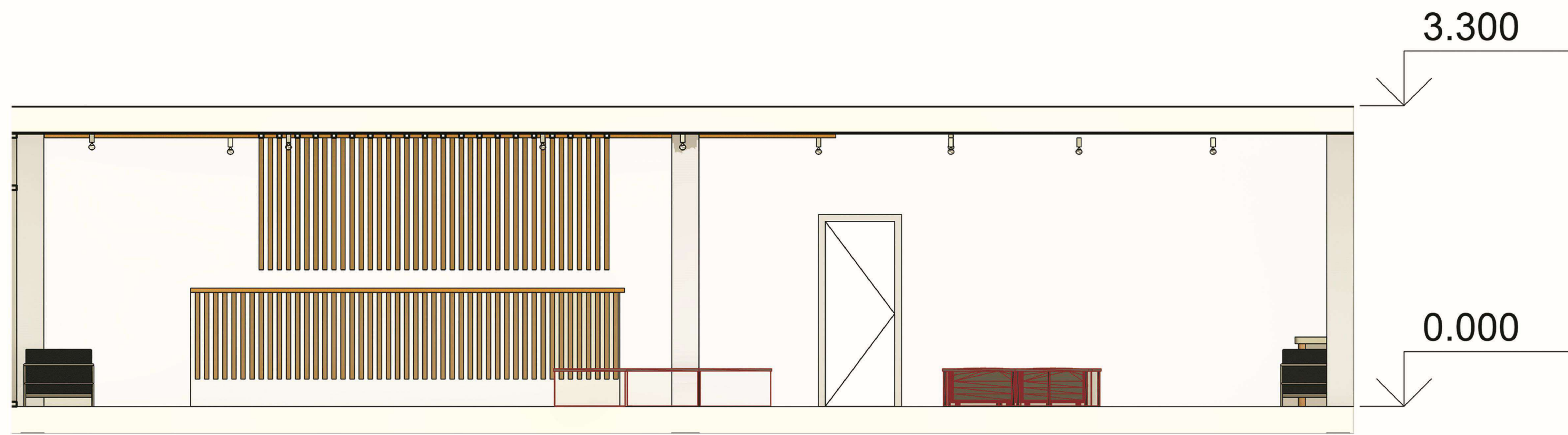
Розгортка по стіні 1-1 М1:50
