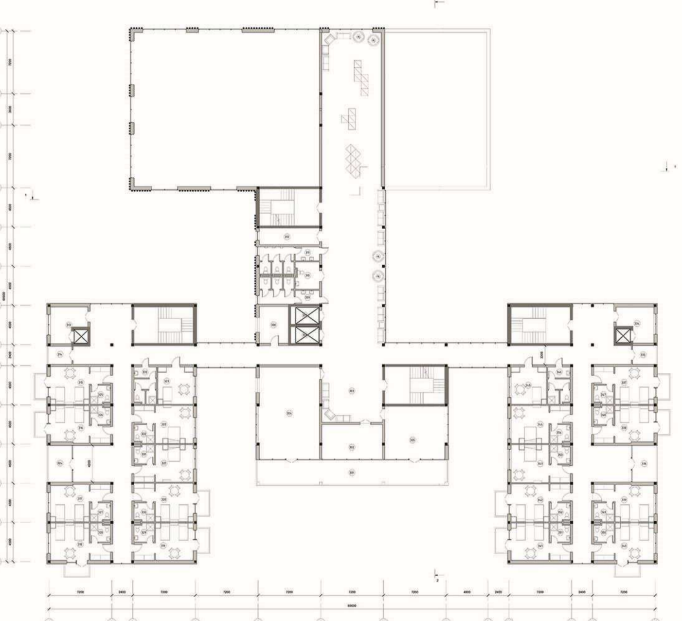
План на відм. +6.600 M1:200
