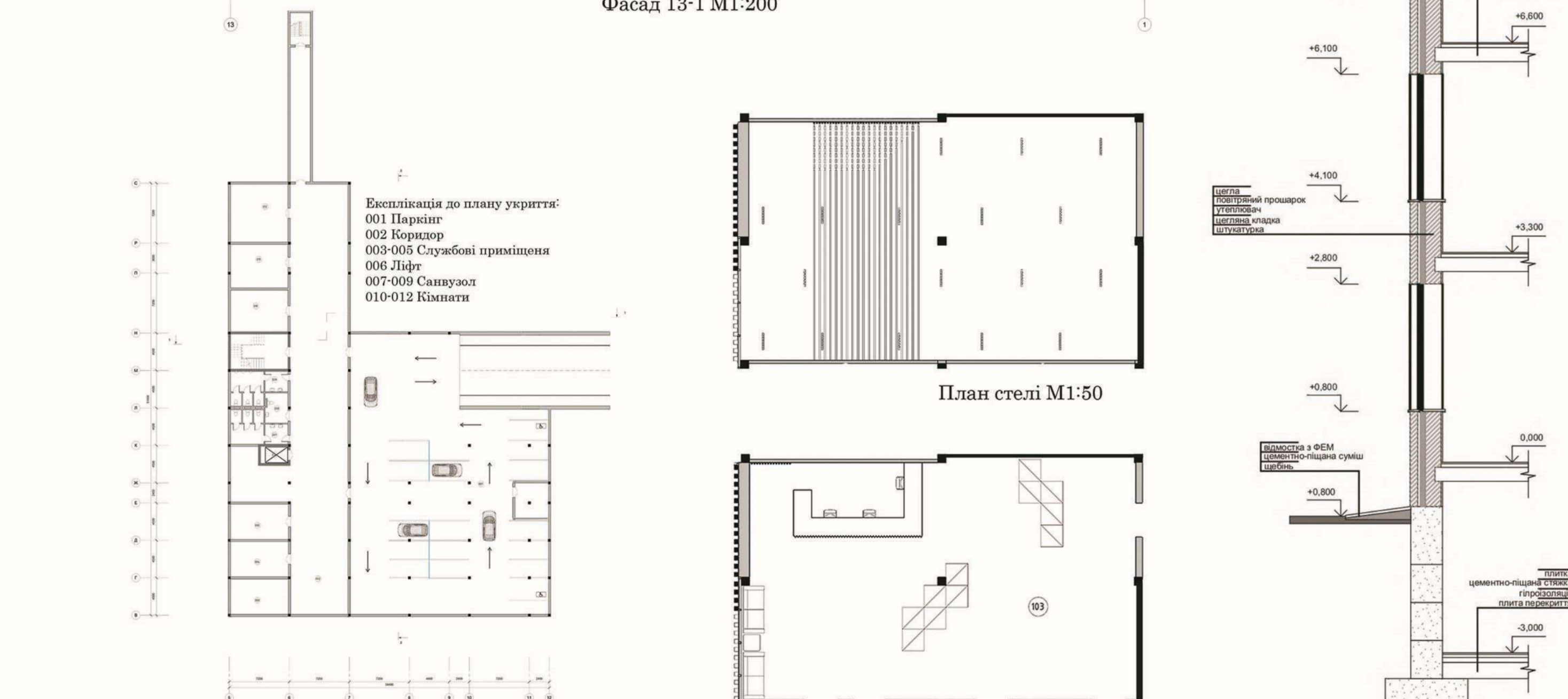
План на відс. -3.300 M1:200
