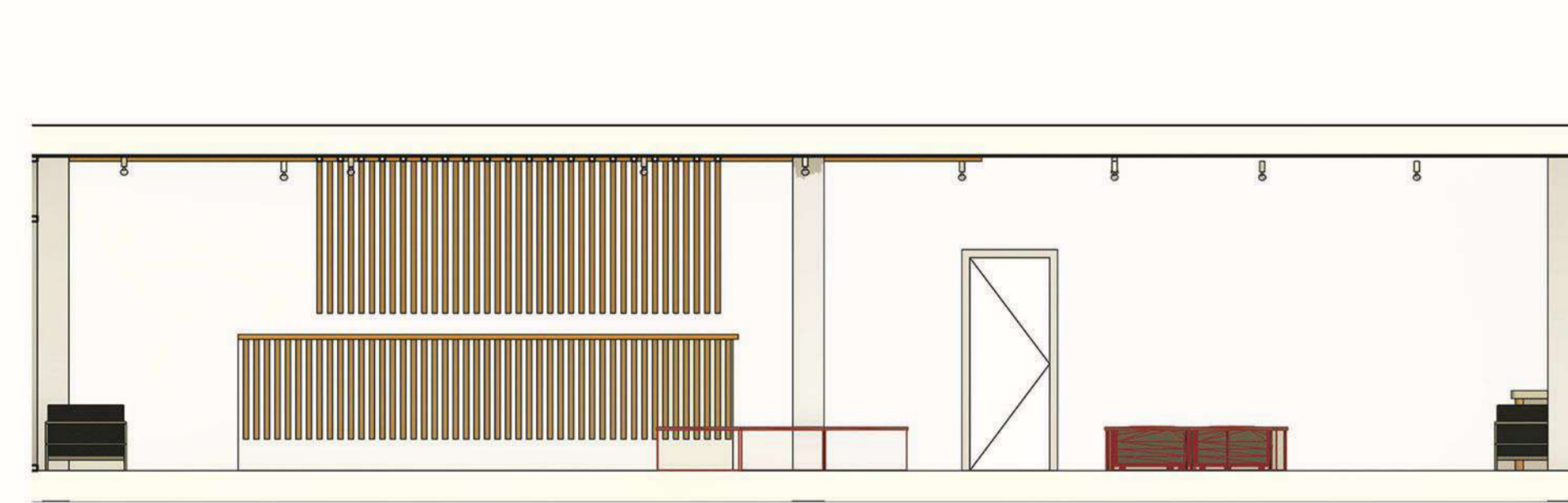
Розріз по стіні 1-1 M1:50
