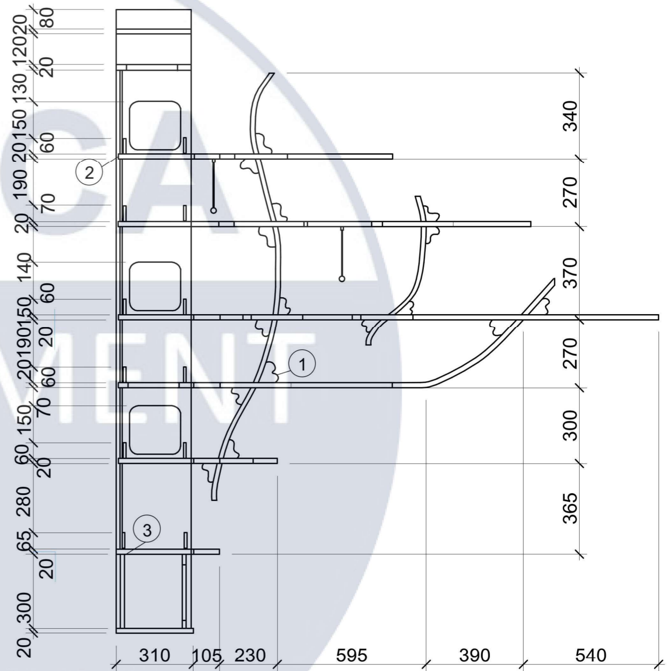
Розріз Б-Б
