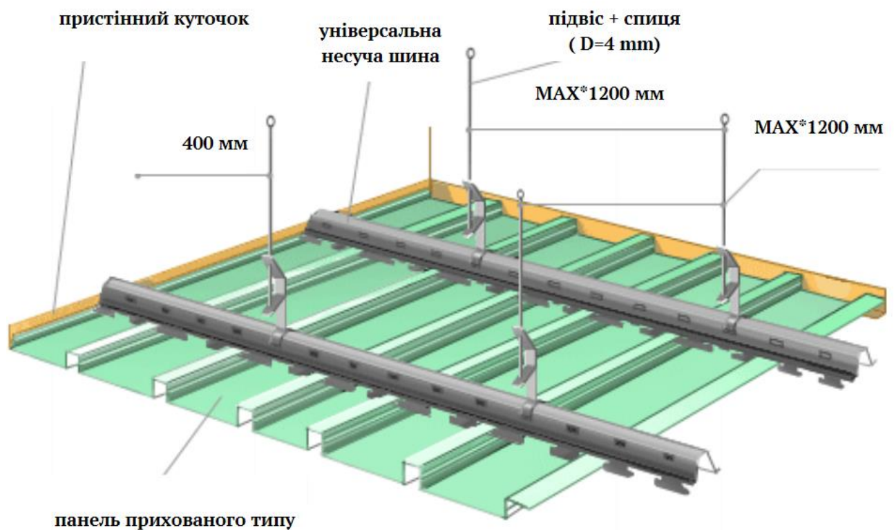
Рис. 4.4. Схема стелі у дитячому закладі.
