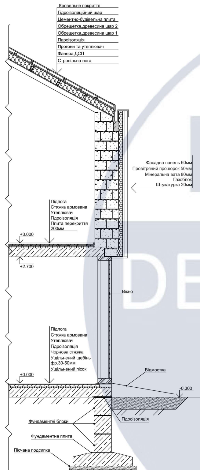
Конструктивний вузел
