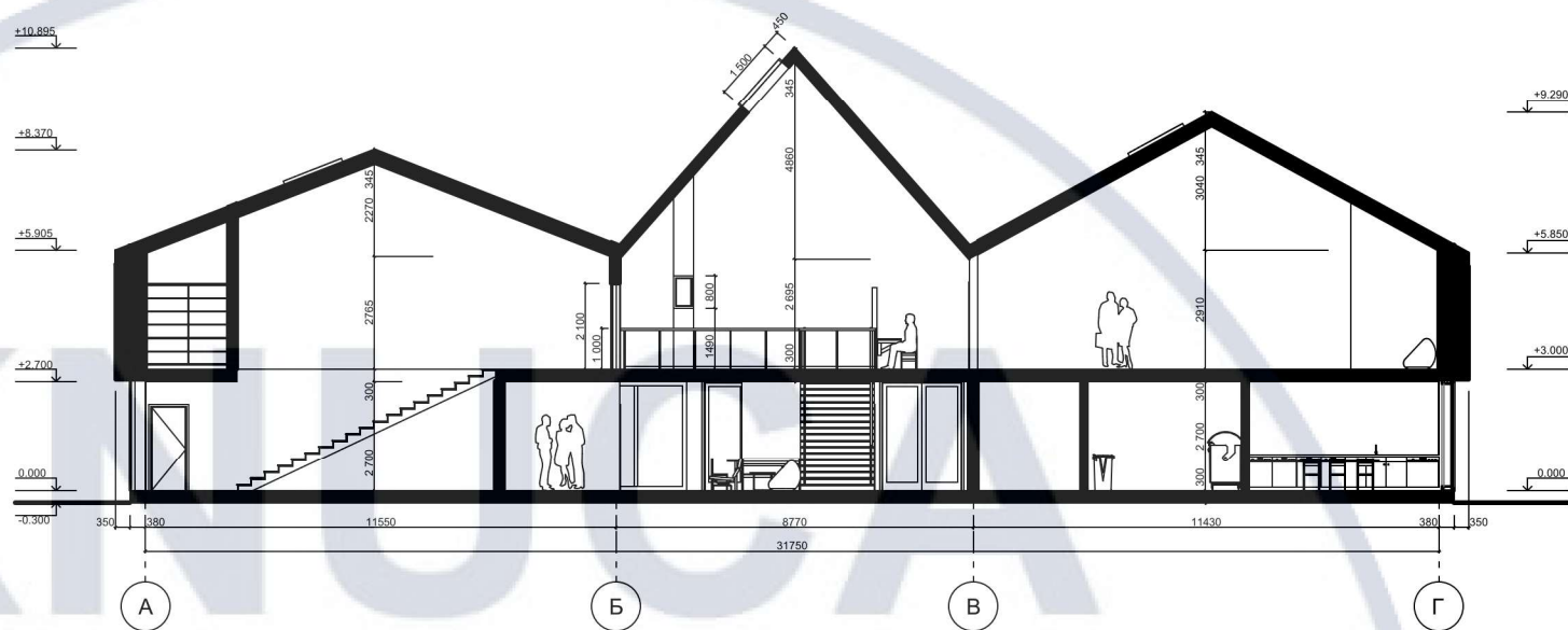
Розріз 1-1
