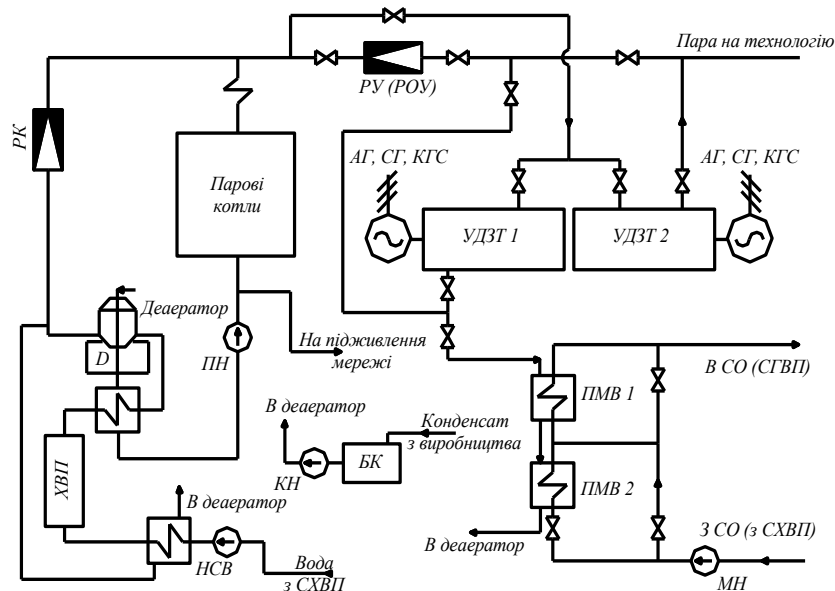
Рис. 1. Принципова схема установки динамічного зниження тиску з електрогенераторами та її місце в системі паропостачання підприємства.
