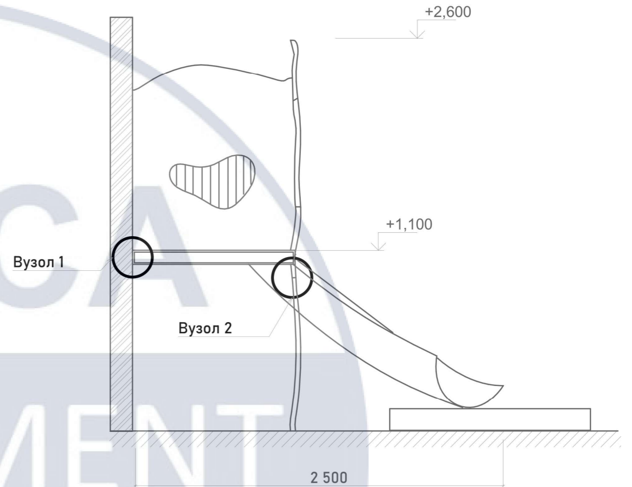
Розріз 1-1
