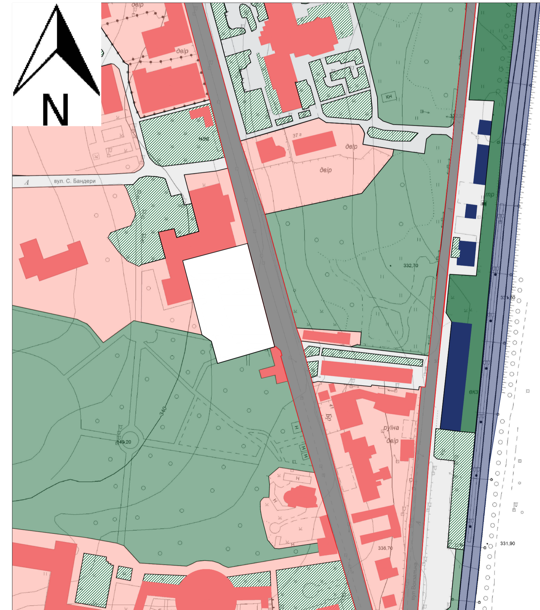
Опорний план М 1:2000
