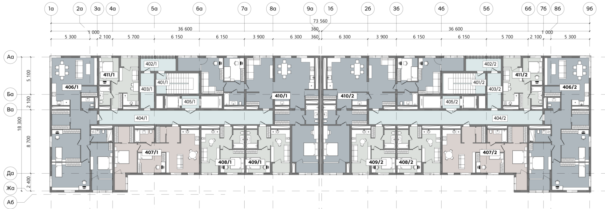
Експлікація приміщень типового поверх житлового блоку №1
