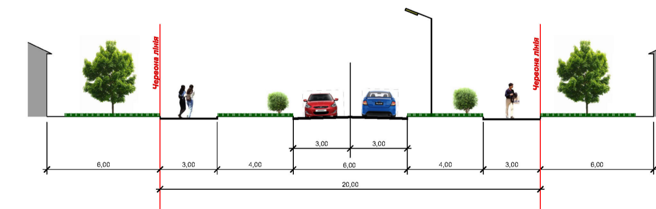
ПРОФІЛЬ ВУЛИЦІ IV-IV
