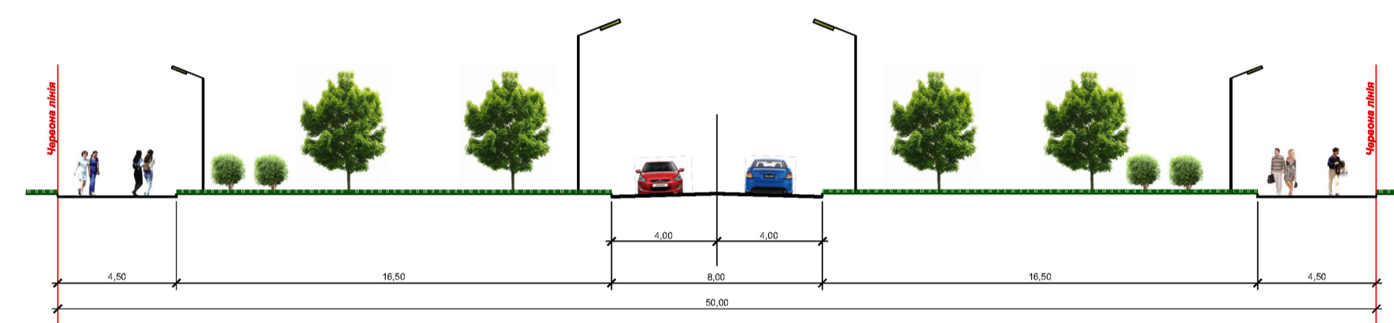
ПРОФІЛЬ ВУЛИЦІ II-II
