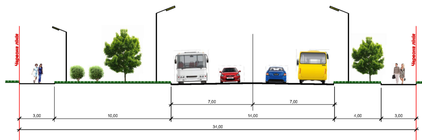
ПРОФІЛЬ ВУЛИЦІ III-III
