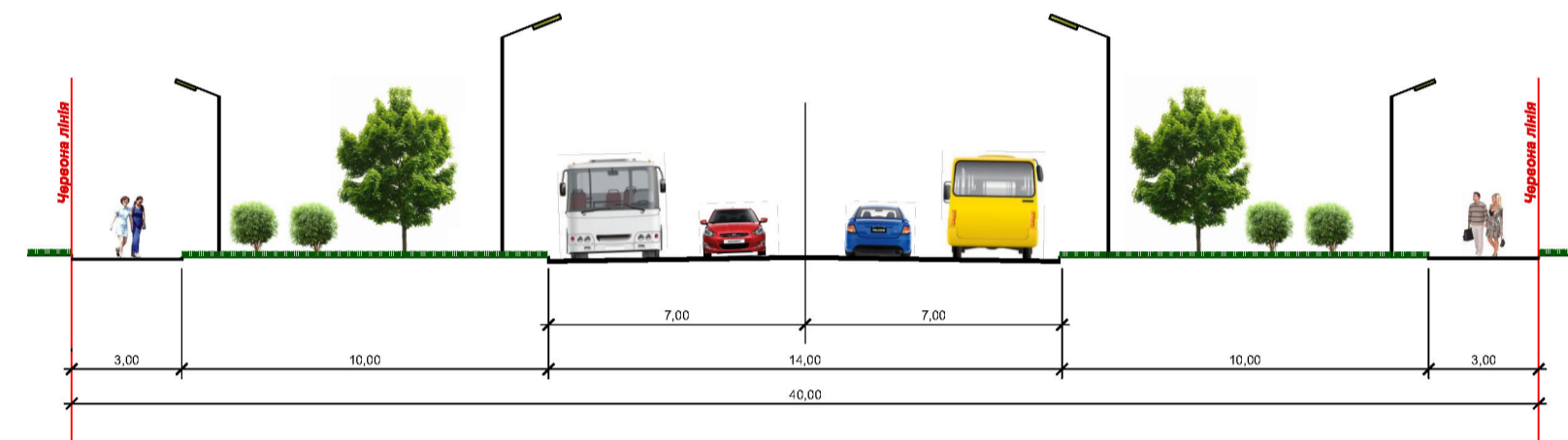
ПРОФІЛЬ ВУЛИЦІ I-I
