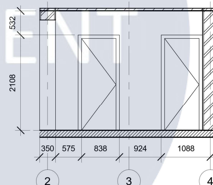
Розгортка 13-14
