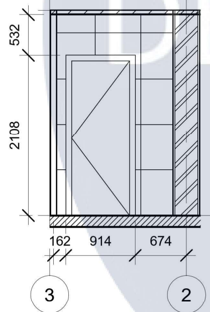
Розгортка 19-20
