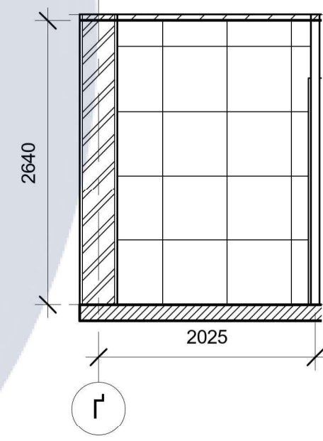
Розгортка 22-19
