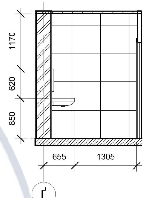
Розгортка 18-15
