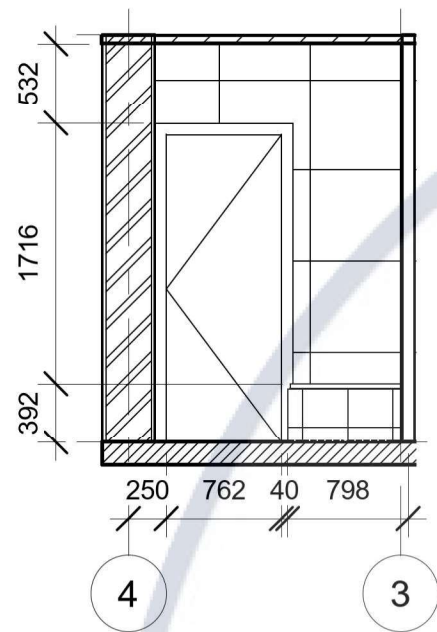
Розгортка 15-16
