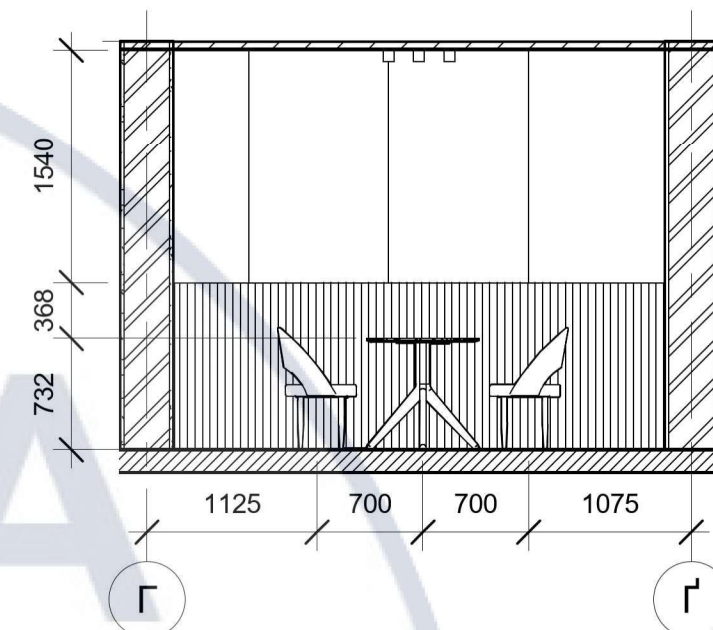
Розгортка 10-11
