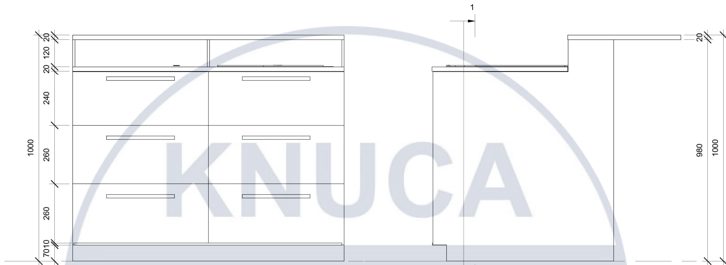
Вид спереду, М1:10
