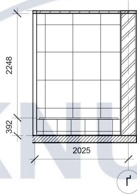
Розгортка 16-17
