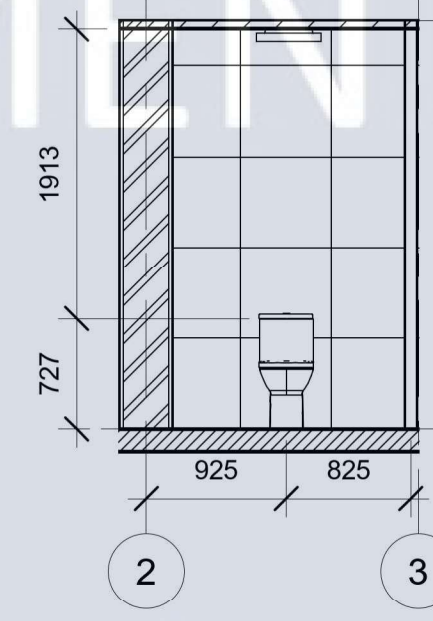
Розгортка 21-22
