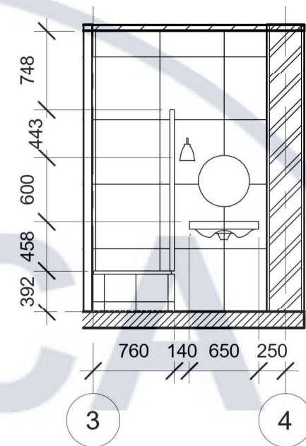
Розгортка 17-18
