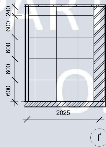
Розгортка 20-21
