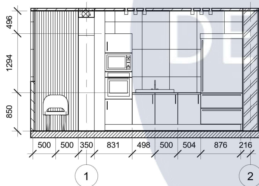
Розгортка 11-12
