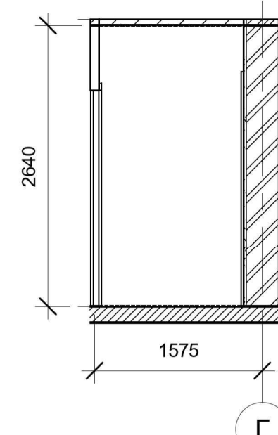
Розгортка 14-9
