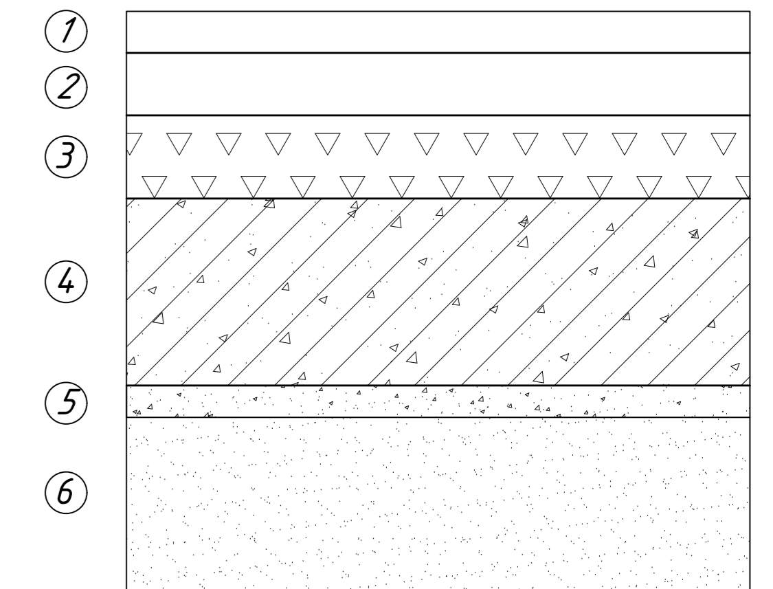
Конструкція дорожнього покриття проїжджої частини
