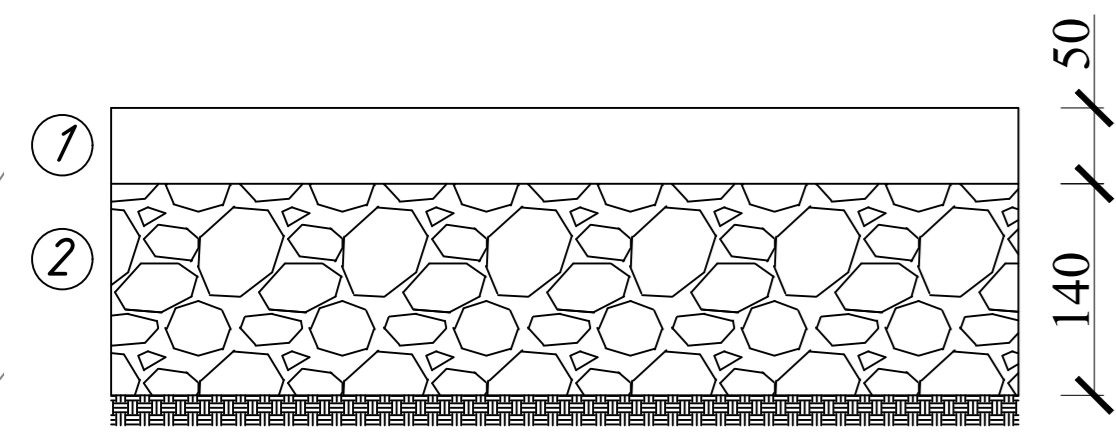
Конструкція тротуару з асфальтобетонним покриттям
