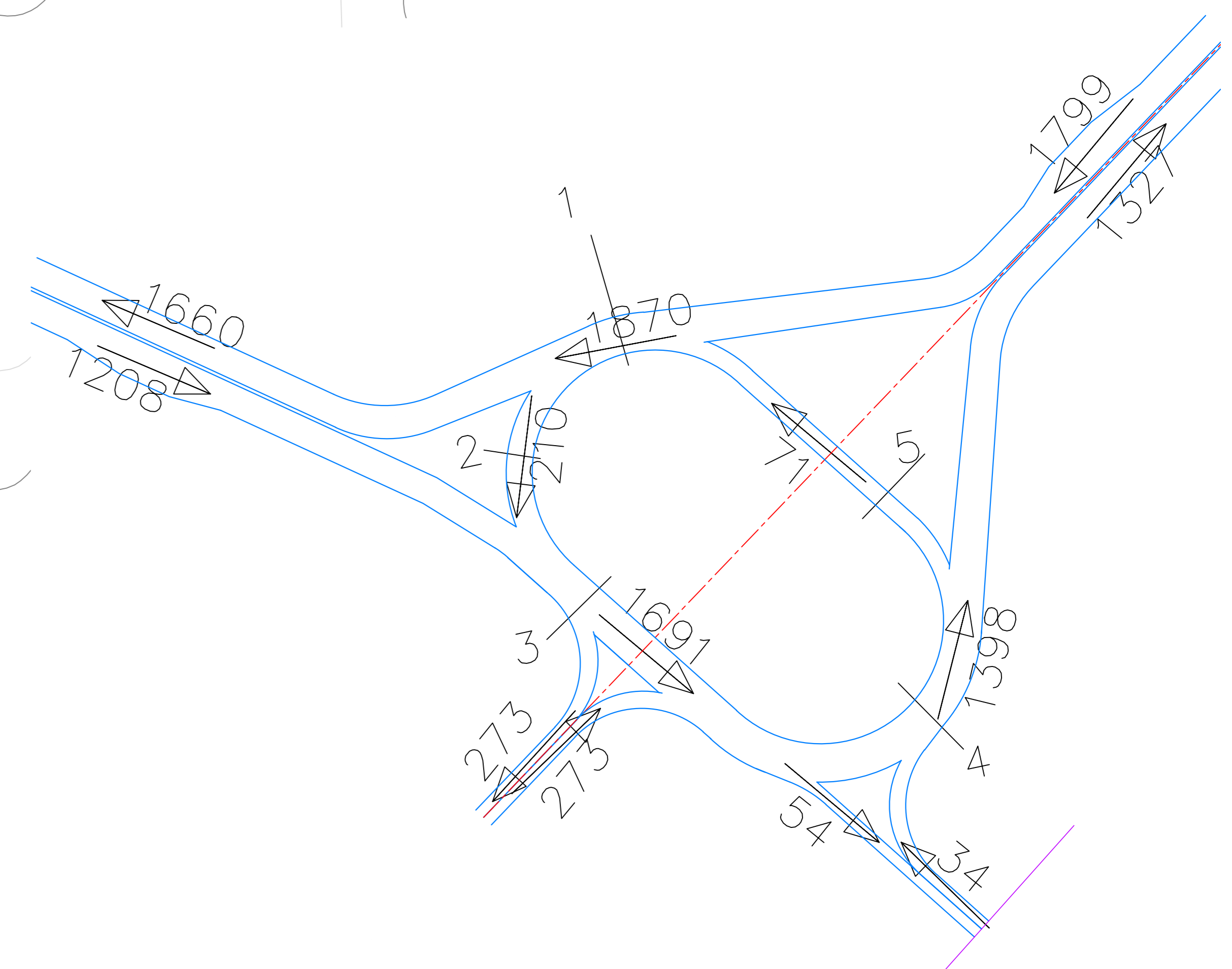
Схема інтенсивності руху транспорту прив. од./год.
