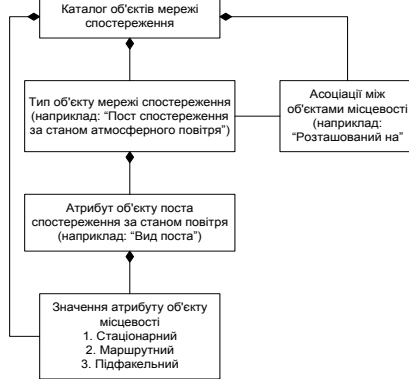
Рис. 4. UML–діаграма загальної принципової схеми каталогу об'єктів мережі спостереження
