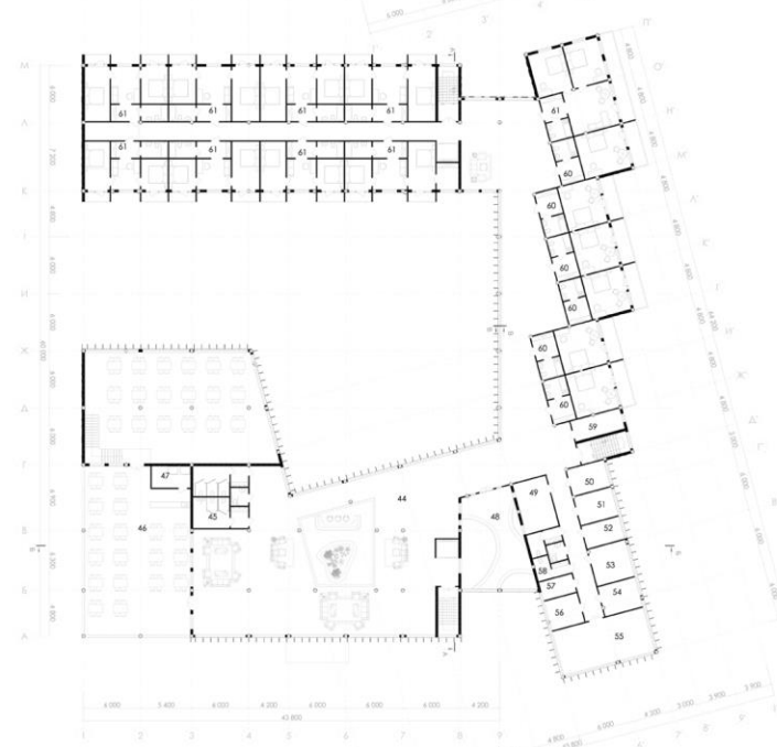
План другого поверху на відмітці +3.300 М1:200
