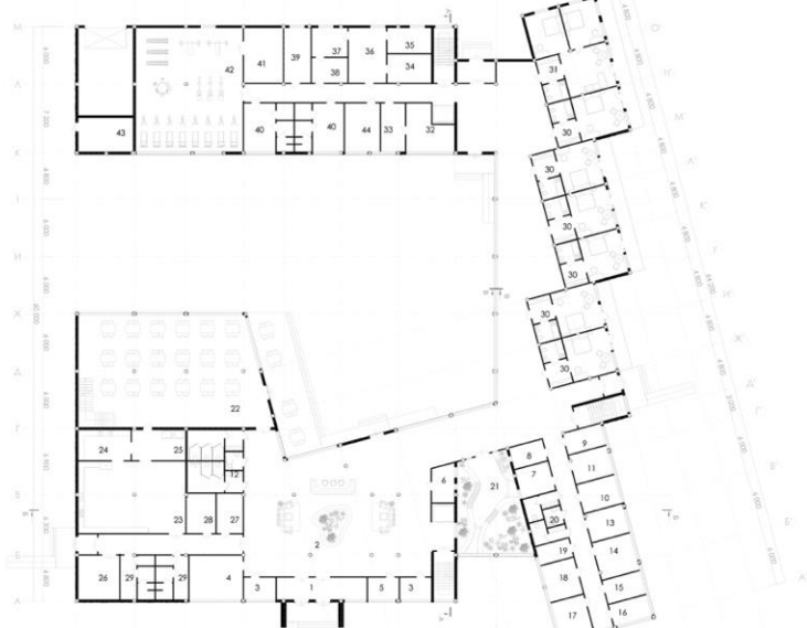
План першого поверху на відмітці 0.000 М1:200
