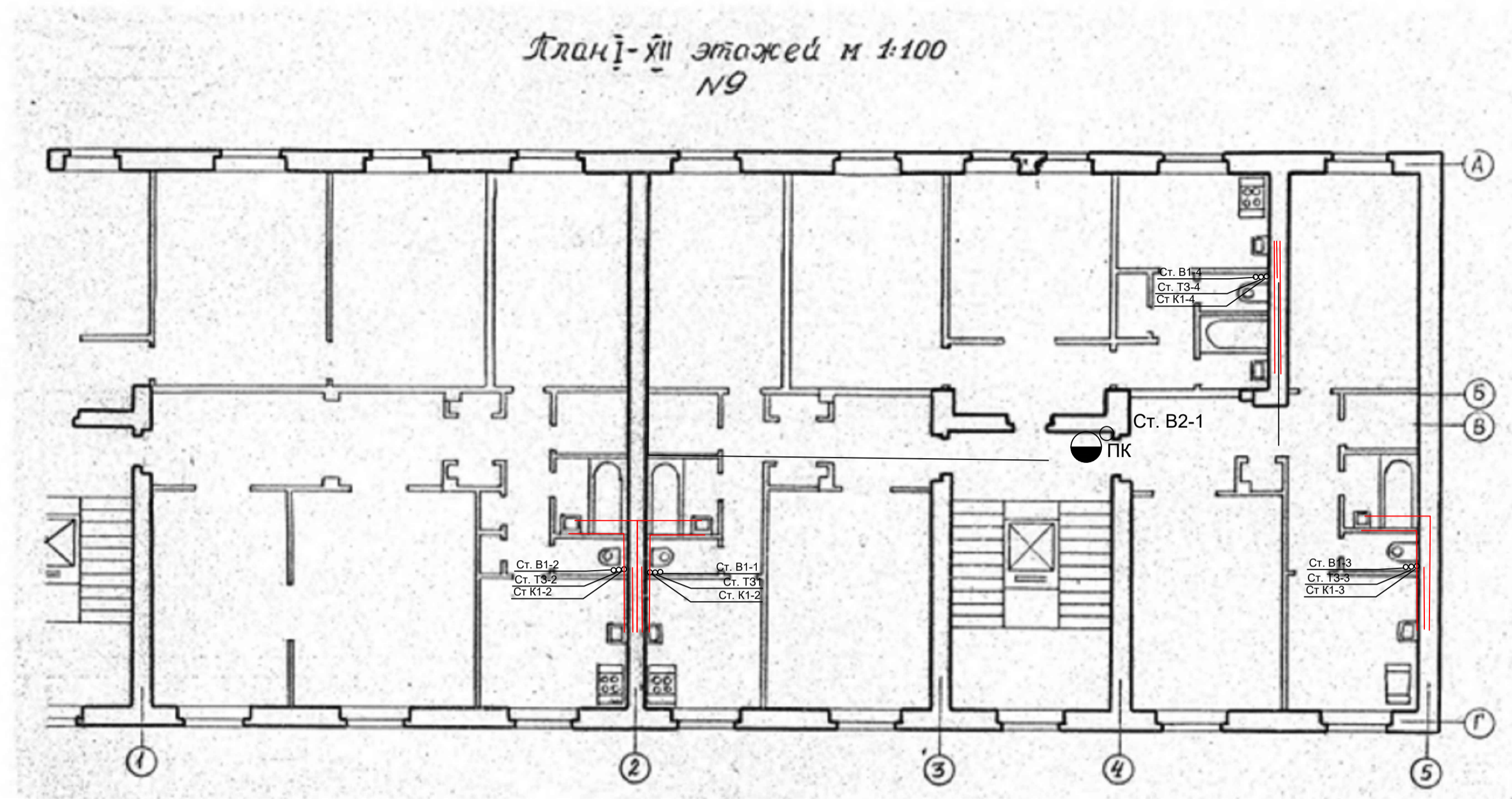
План типового поверху
