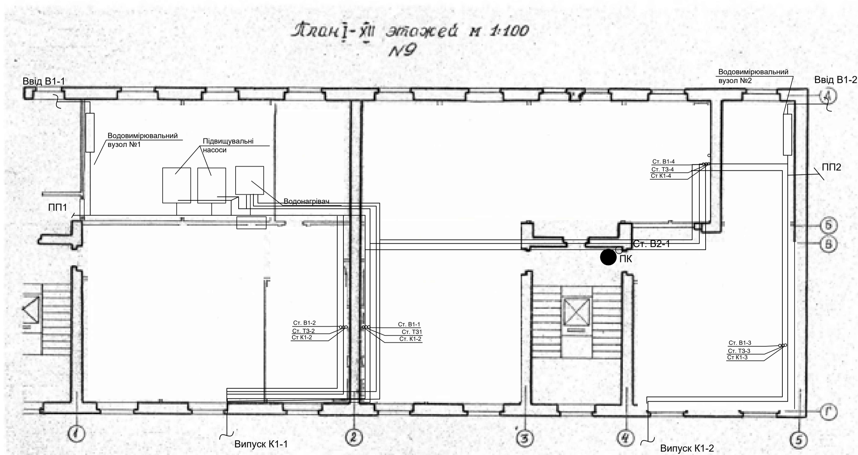
План підвалу
