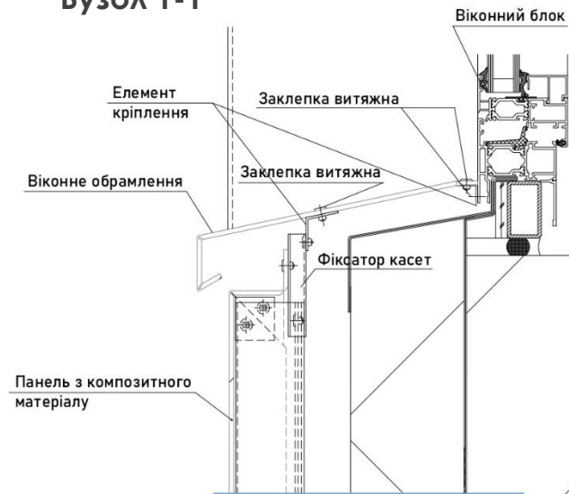
Вузол 1-1
