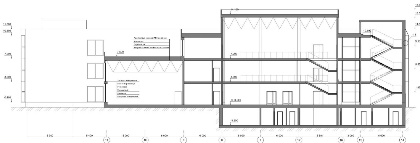
Розріз 2-2
