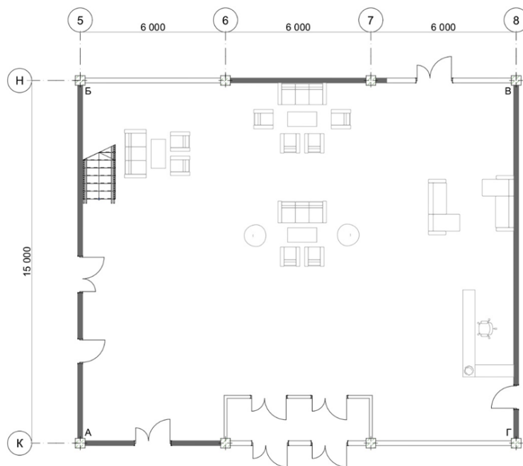
План підлоги і меблів
