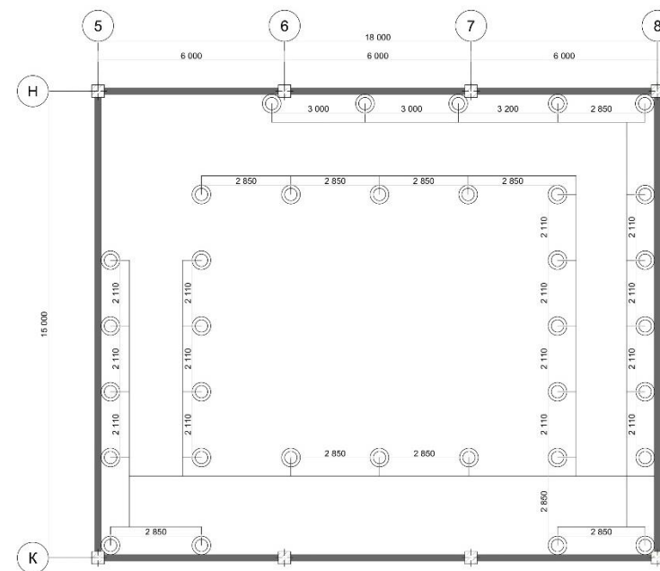
План стелі
