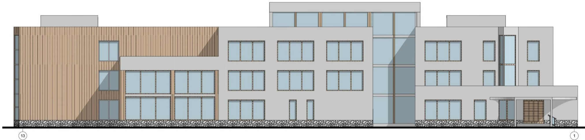
Фасад у вісях 13-1:
