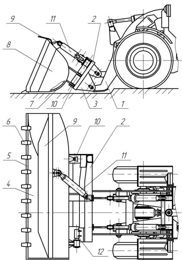
Рис. 1. Ківш навантажувача з боковим розвантаженням: 1 – стріла; 2 – опорна рама; 3 – провухина; 4 – днище; 5 – ріжуча кромка; 6 – зуб; 7, 8 – задня та бічна стінки; 9 – козирок; 10 – шарнір; 11 – гідроциліндр; 12 – фіксатор
