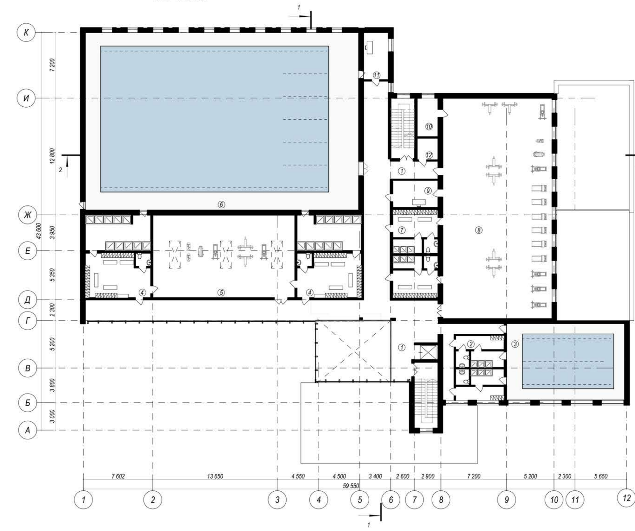
Експлікація 2 поверку:
