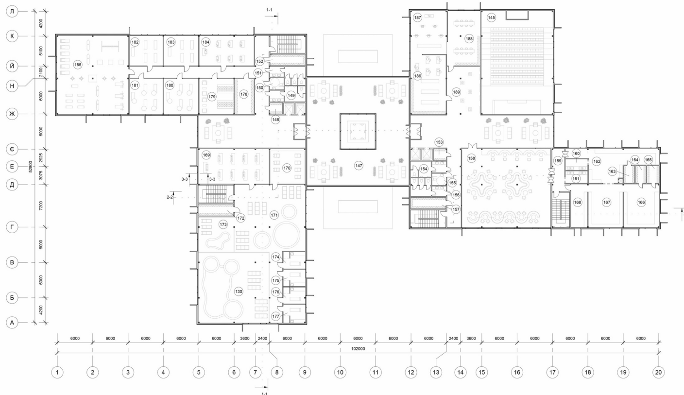
План на відмітці +3.600
