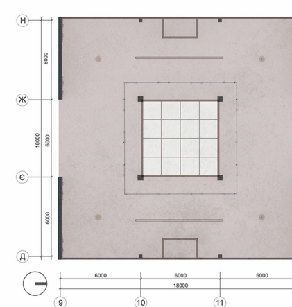
План стелі з розміщенням освітлювальних приладів
