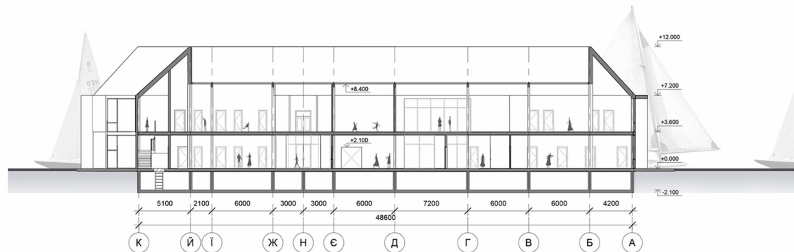
Розріз 1-1
