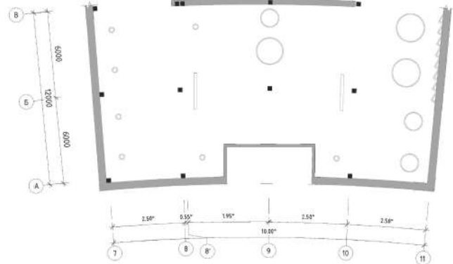
План стелі із освітлення
