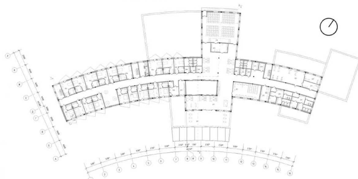
План поверху на відмітці +5.800
