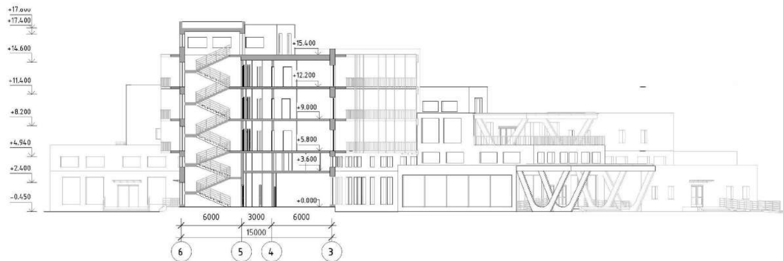
Розріз 1-1
