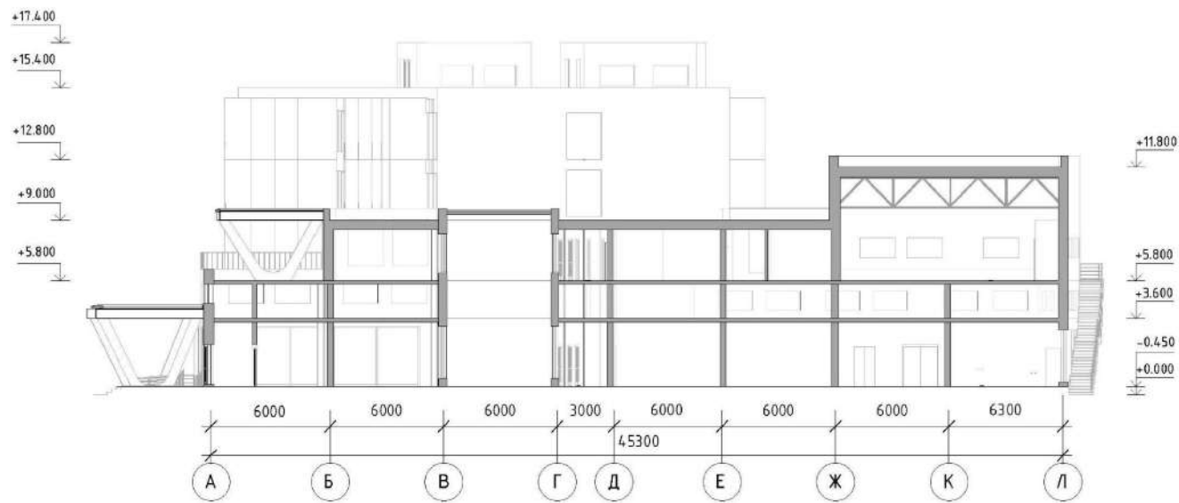
Розріз 2-2
