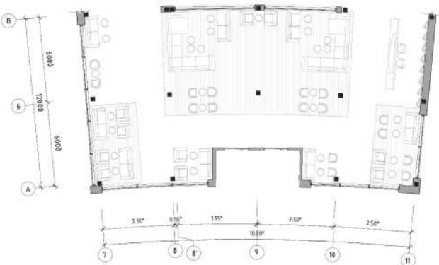
План підлоги із розміщенням обладнання
