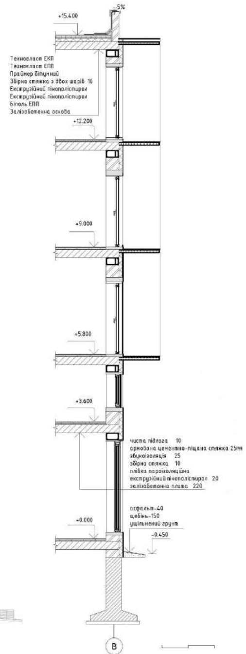
Розріз 3-3
