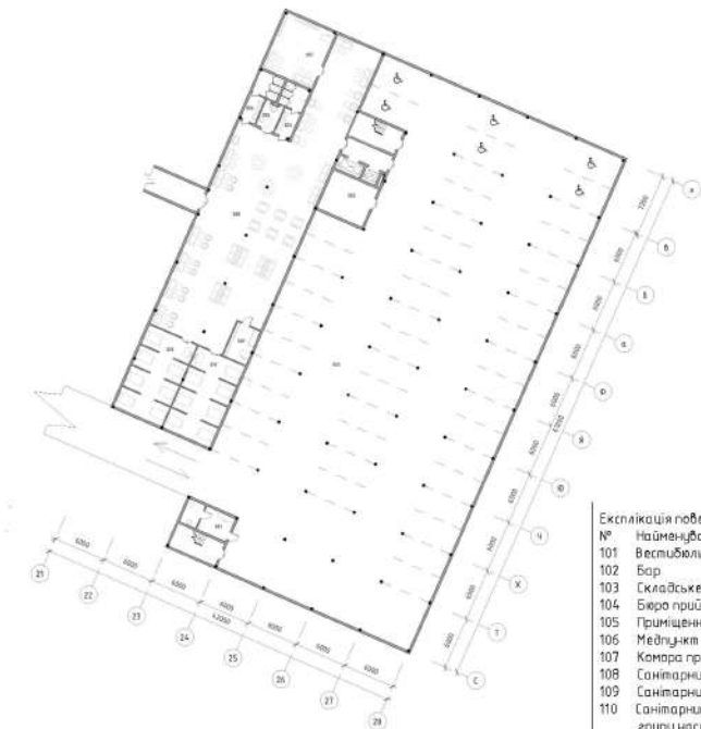
План поверху на відмітці -3.000
