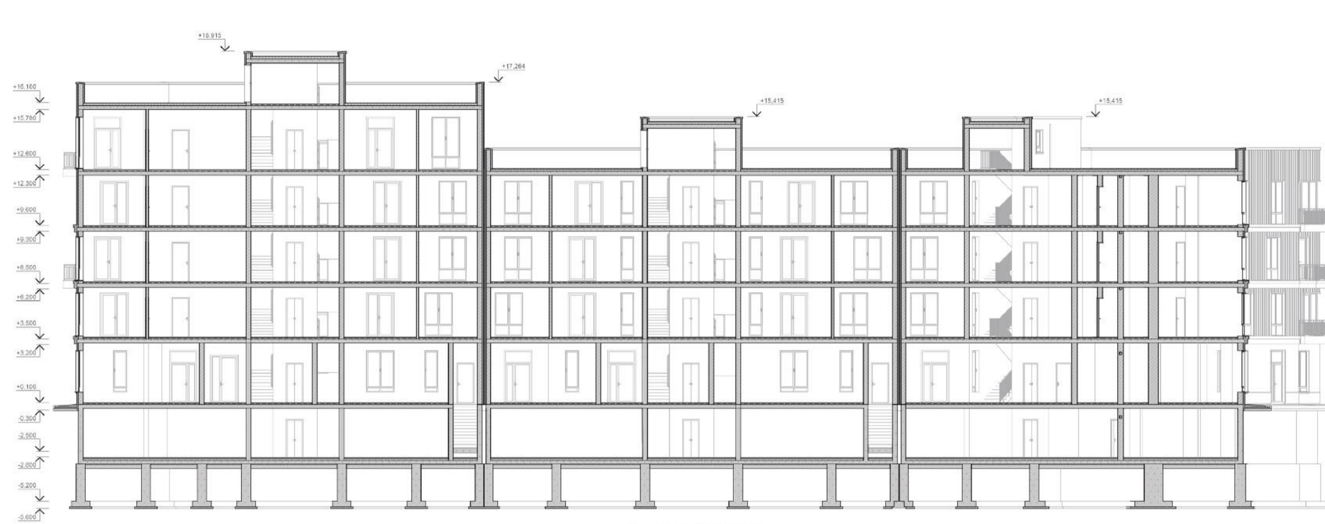
Розріз 2-2 М 1:100
