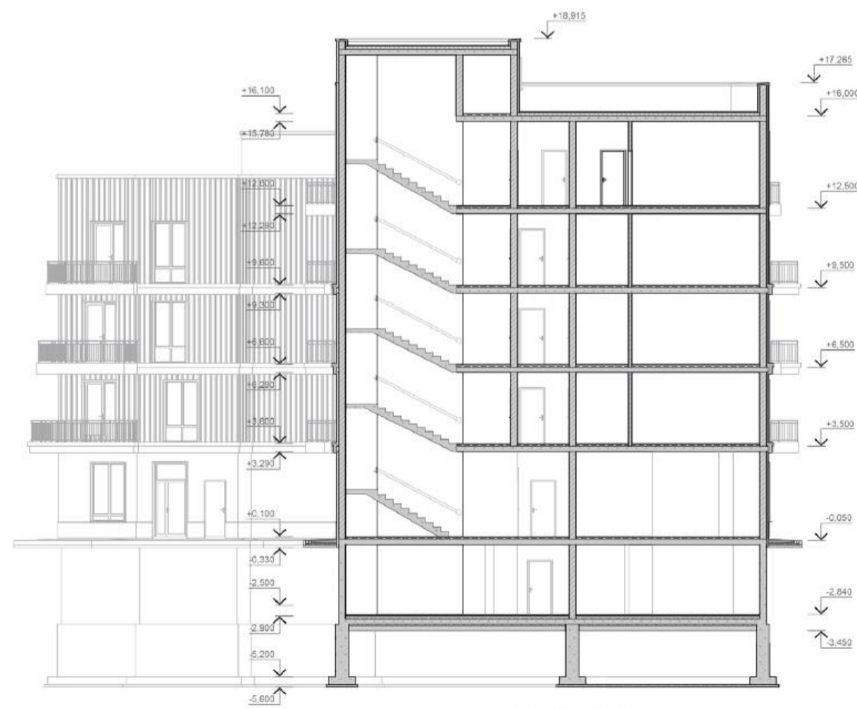
Розріз 1-1 М 1:100
