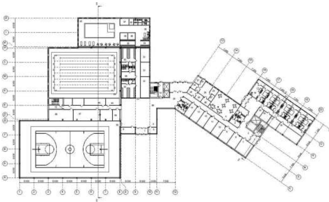
План 1 поверху
