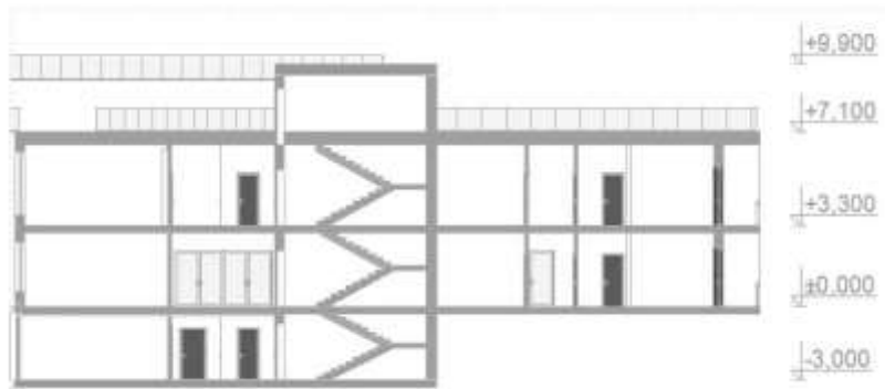
Розріз 2-2
