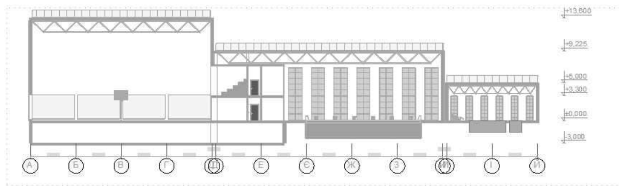
Розріз 1-1
