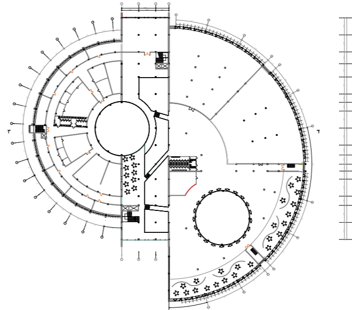
План 2-го поверху
