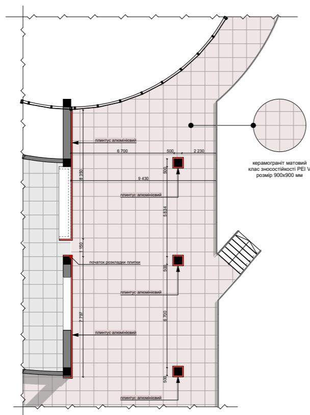
План підлоги
