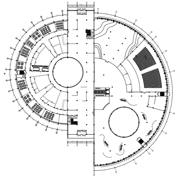
План 1-го поверху
