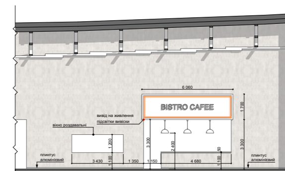
Розгортка
