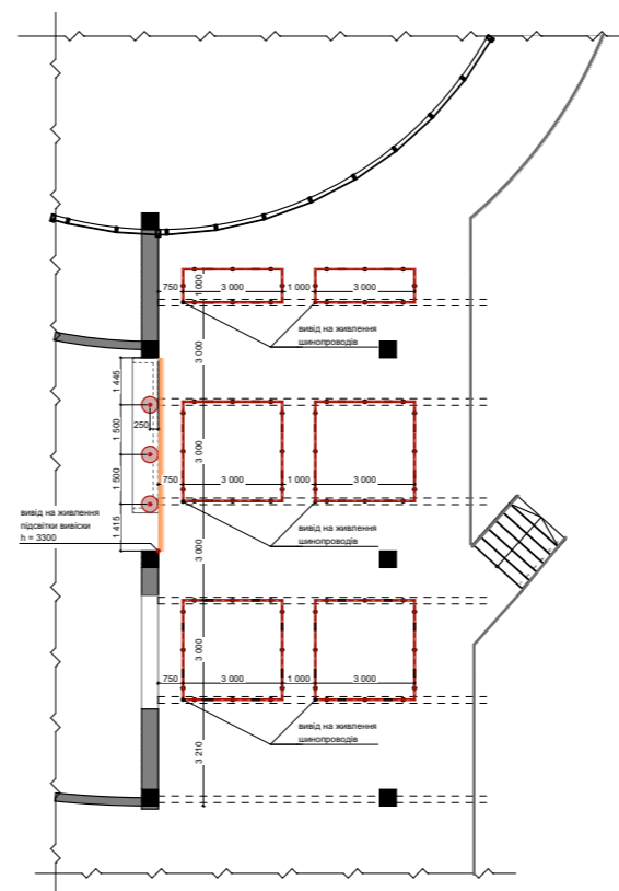
План стелі
