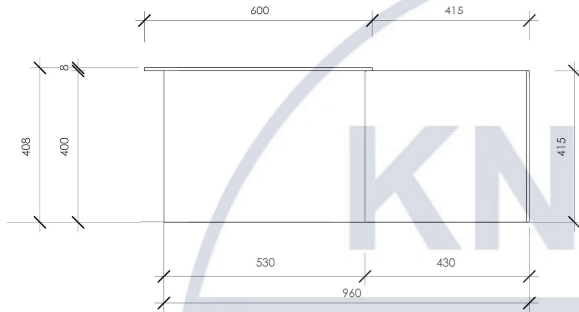
Вид спереду М 1:10
