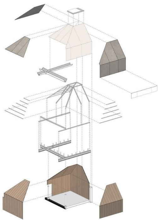
Схема влаштування покрівлі
