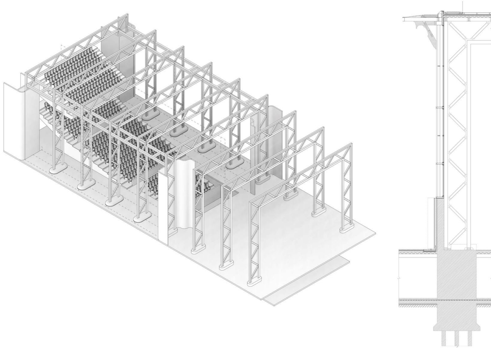
Конструктивні рішення
