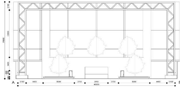
Розгортка А-Г
