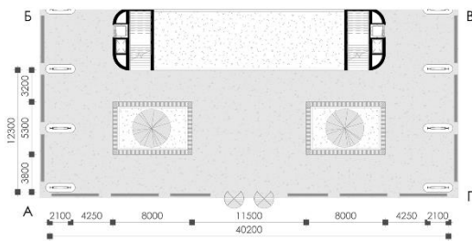
План підлоги
