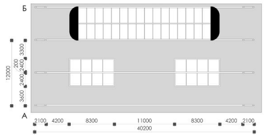
План стелі
