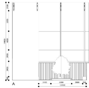
Розгортка А-Б
