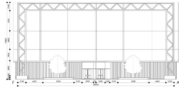
Розгортка Г-А
