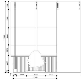
Розгортка Г-В
