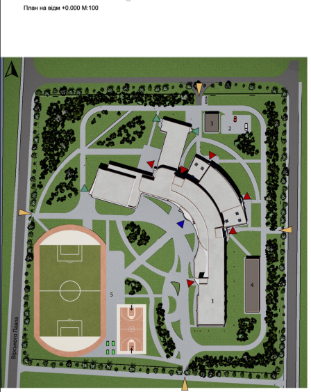
Генеральний план М:500
