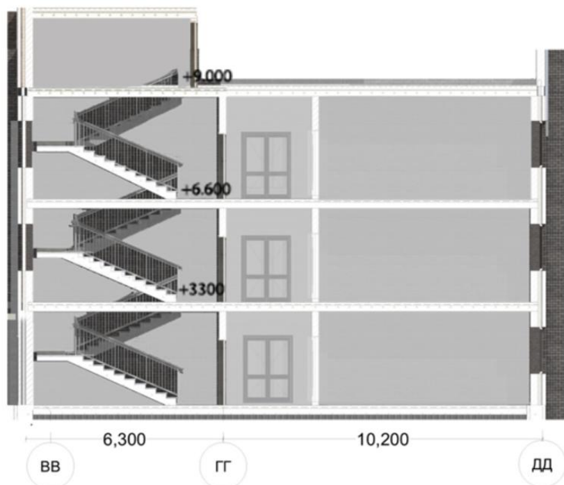
Розріз 1-1 М:200
