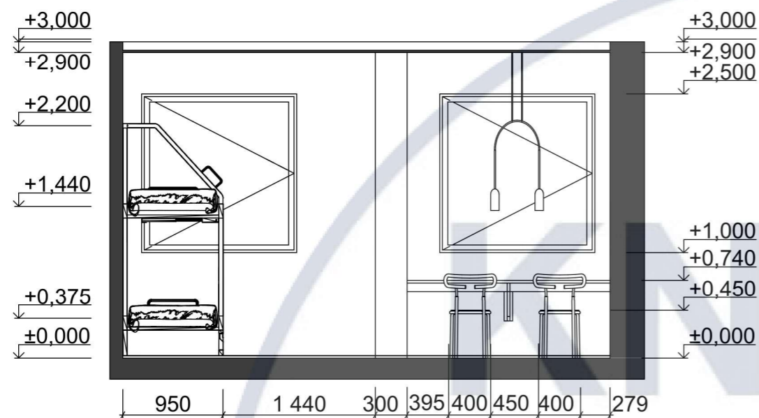
Розгортка 1-2
