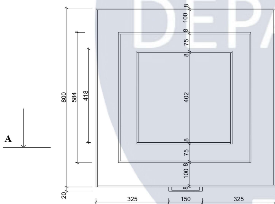
Вид зверху
