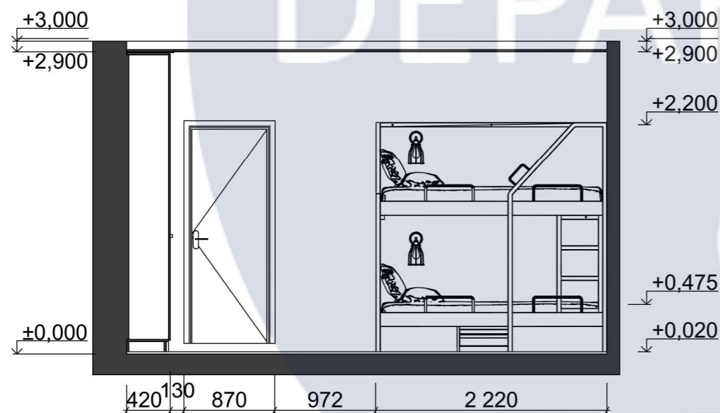
Розгортка 3-4
