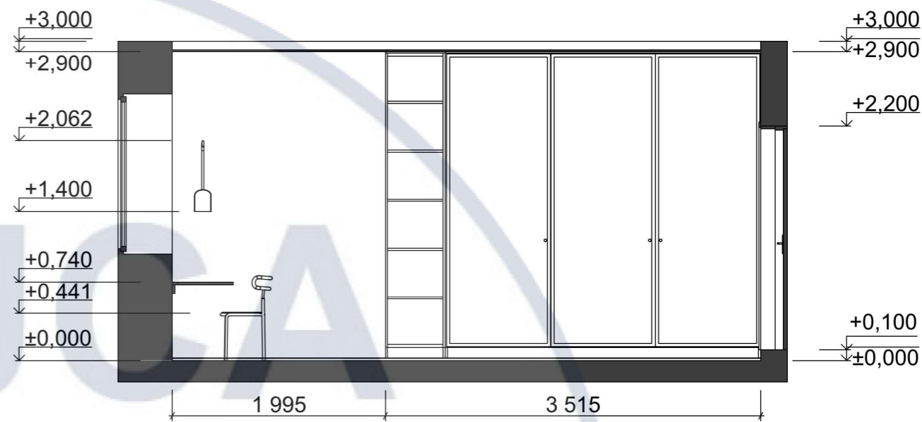
Рзгортка 2-3
