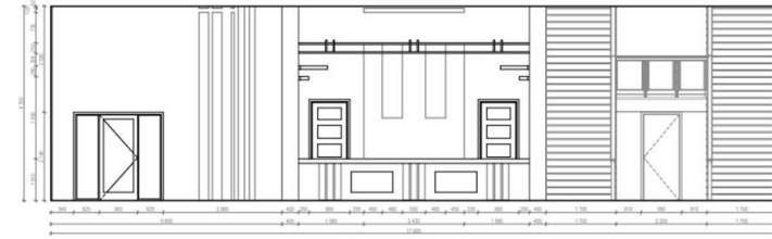
Розгортка А-Б
