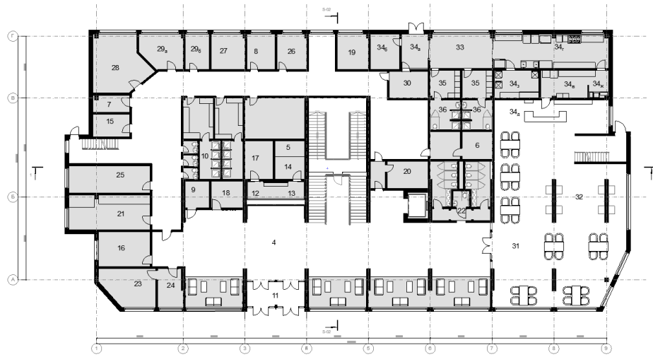
План 1 поверху
