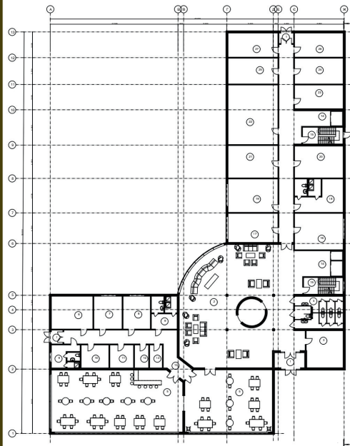
План поверху на відмітці 0.000 M 1:100
