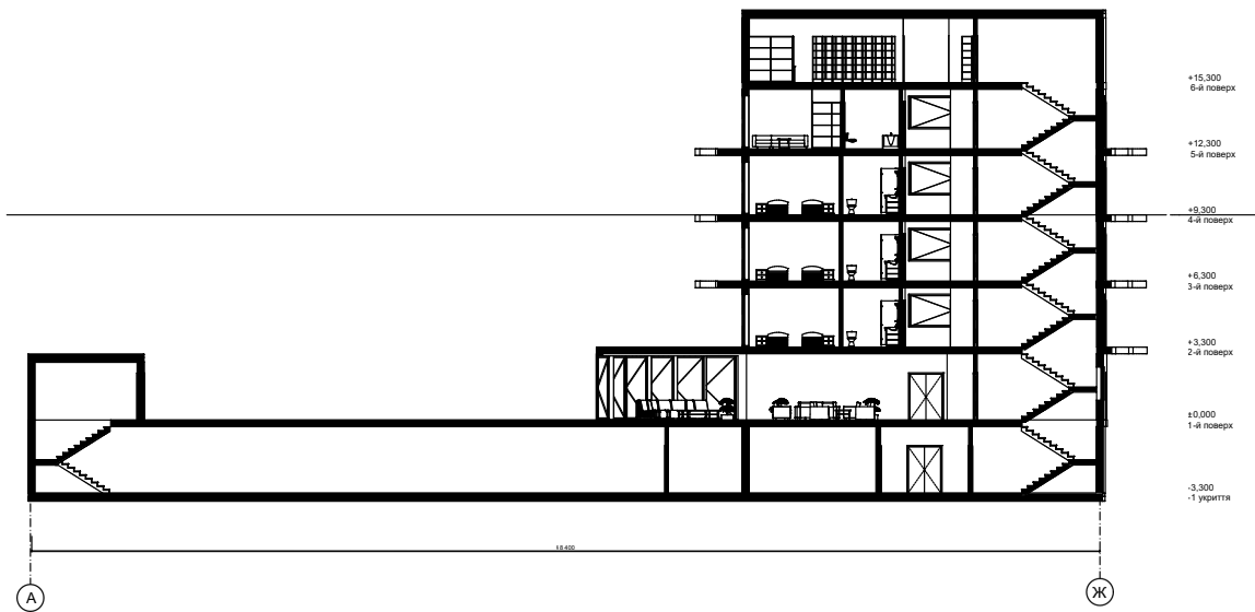
Розріз А-Ж М 1:200
