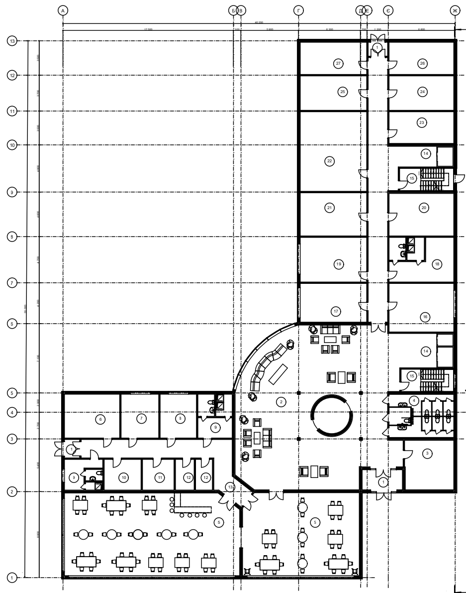
План поверху на відмітці 0.000 М 1:100
