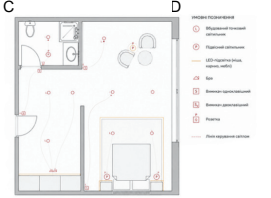
План стелі m 1:200
