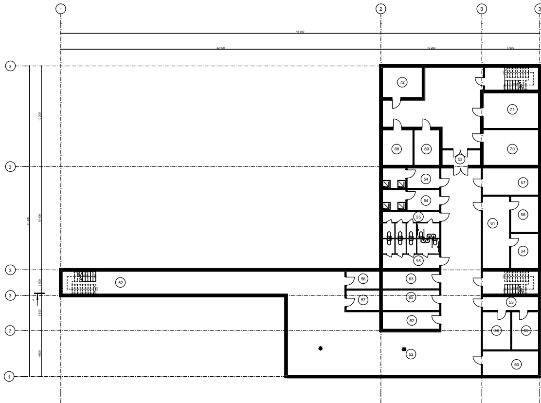
План поверху на відмітці -3.300 М 1:100
