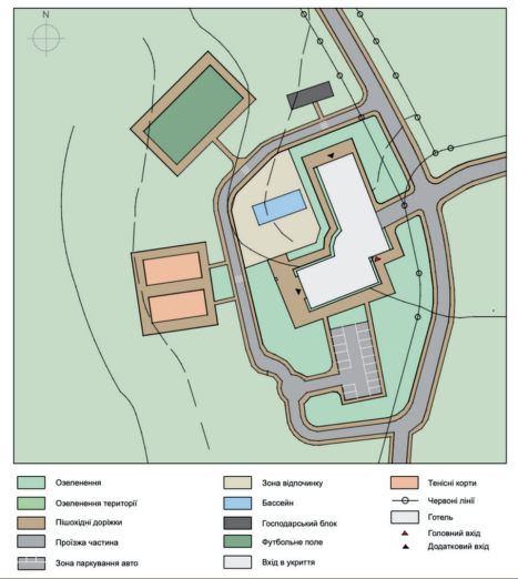
Генеральний план M 1:500
