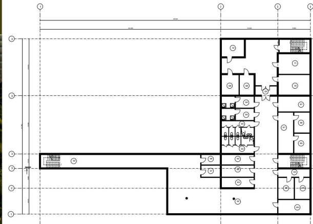
План поверху на відмітці -3.300 M 1:100
