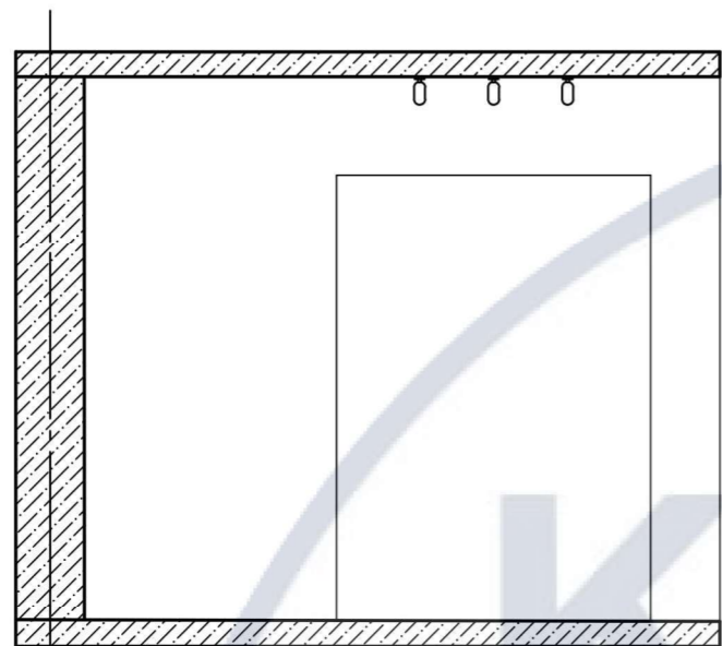
Розгортка 28-29 М1:50
