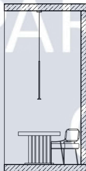
Розгортка 33-34 М1:50
