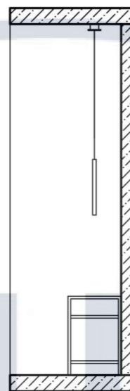
Розгортка 29-30 М1:50
