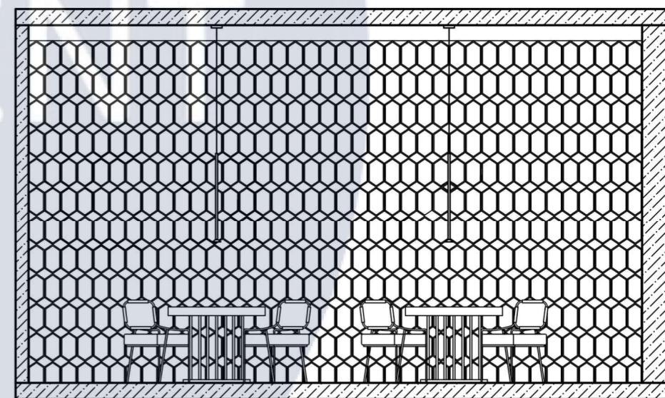
Розгортка 34-35 М1:50
