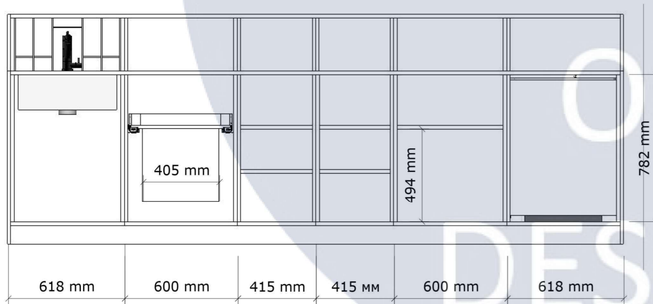
Вид ззаду без фасадів М1:20
