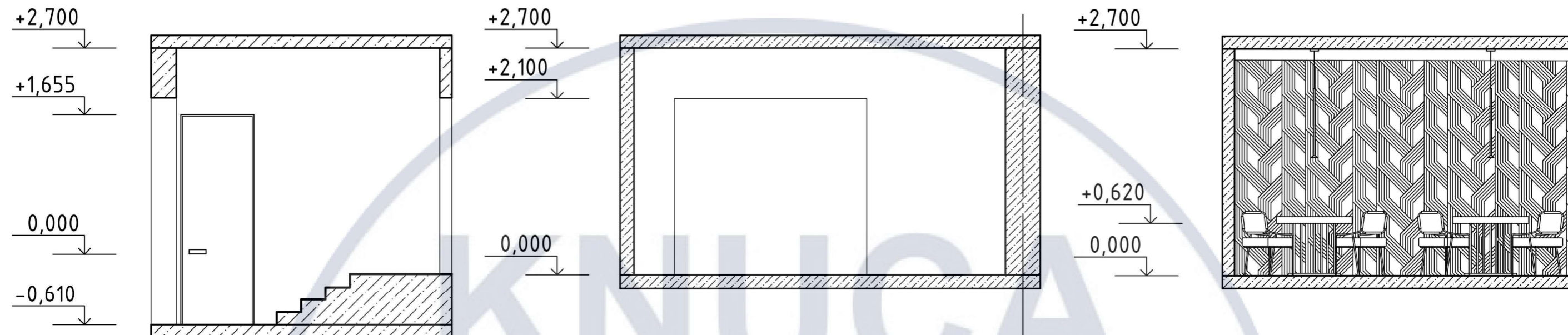
Розгортка 36-37 М1:50
