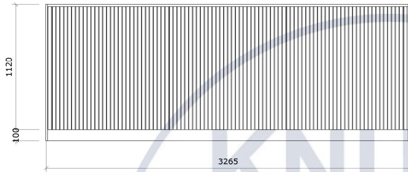
Вид спереду М1:20
