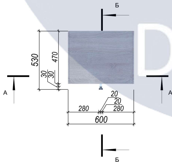
Вид зверху, М 1:20
