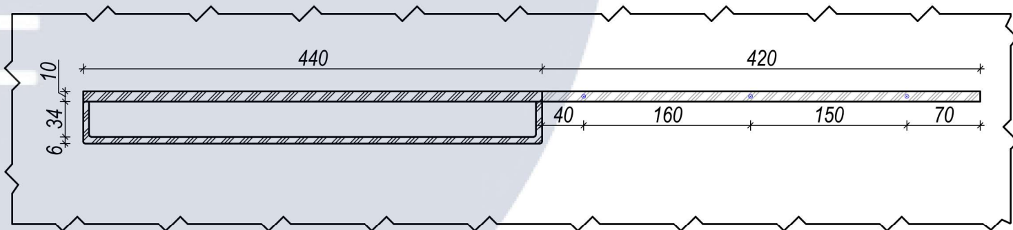
Вузол 2, М 1:5 Вішалка поперечна з доводчиком
