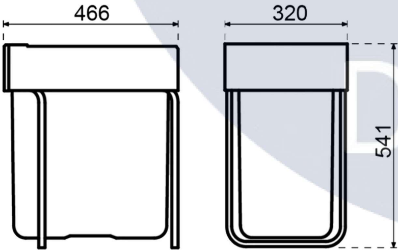
Габаритні розміри вставного відра для сміття
