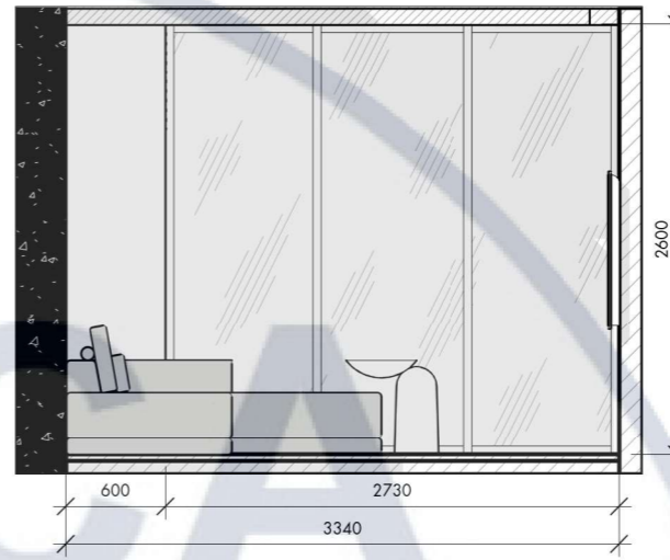
Кухня-вітальня 3 1 : 50
