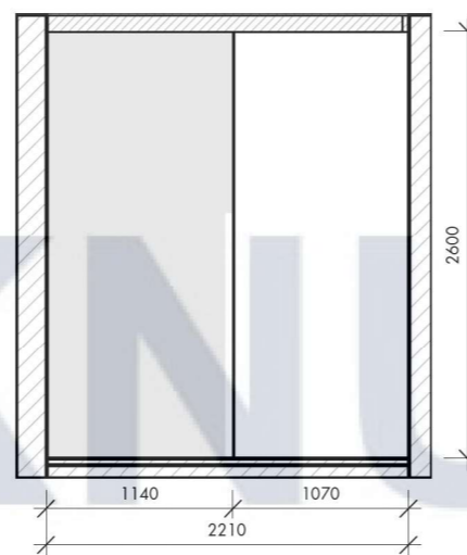
Коридор 2 1 : 50
