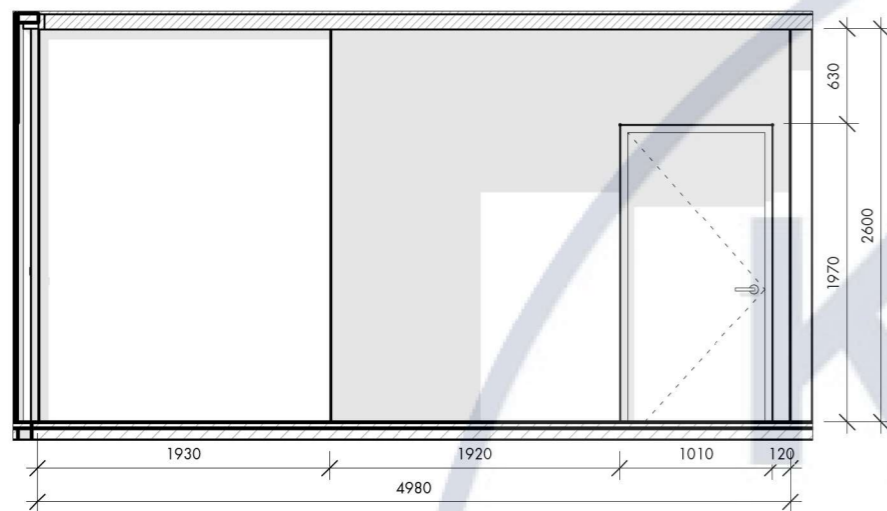
Коридор 1 1 : 50
