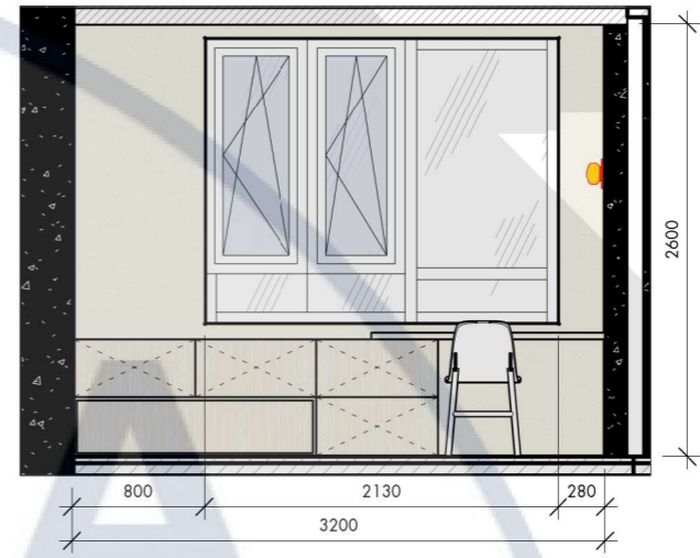
Кабінет 4 1 : 50
