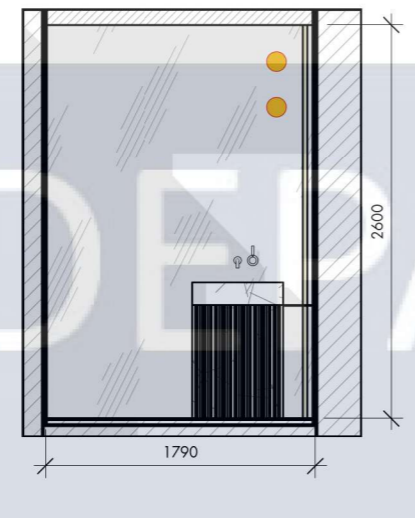
Санвузол 2 1 : 50
