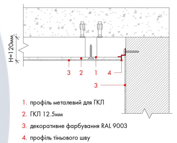
Розріз 1 (тіньовий шов)
