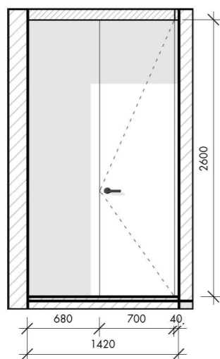
Гардеробна 1 1 : 50
