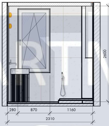
Санвузол 3 1 : 50
