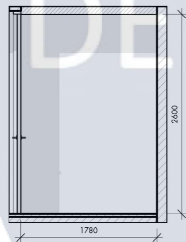
Гардеробна 2 1 : 50
