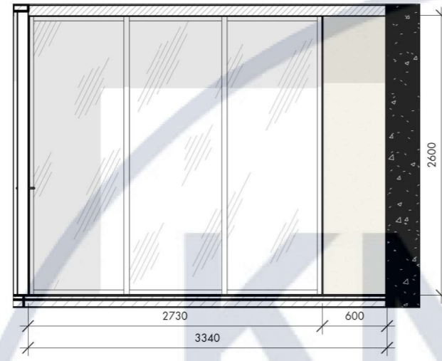
Кабінет 2 1 : 50
