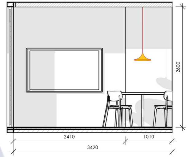
Кухня-вітальня 4 1 : 50
