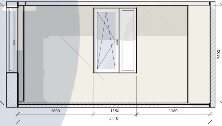
Дитяча 4 1 : 50
