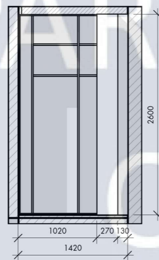
Гардеробна 3 1 : 50
