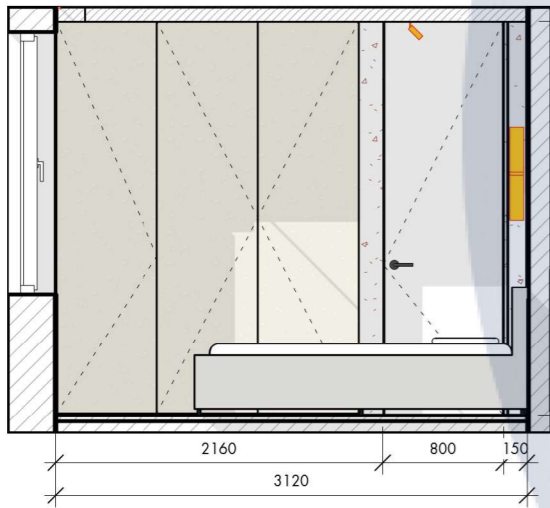
Дитяча 1 1 : 50
