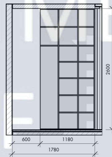
Гардеробна 4 1 : 50
