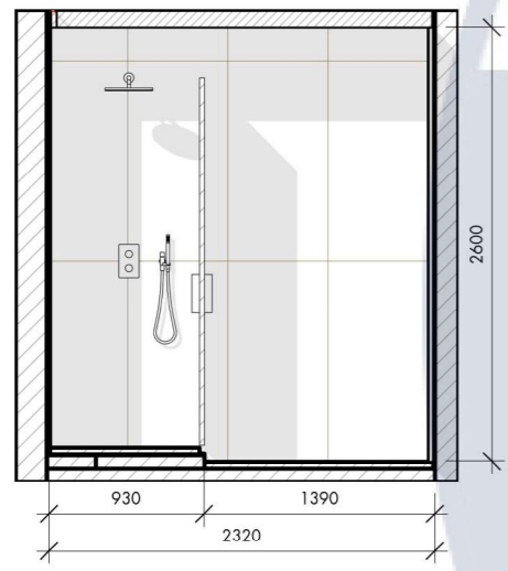
Санвузол 1 1 : 50
