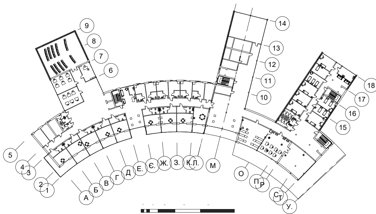
План второго поверху
