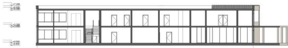
Розріз в осях 18-1 М1:100
