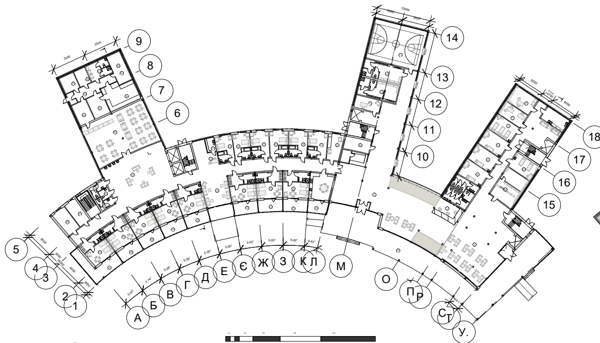
План первого поверху
