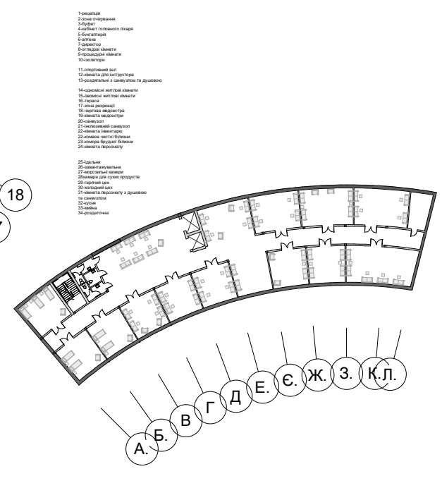
План укріття
