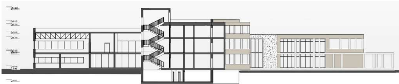
Розріз в осях 9-1 М1:100
