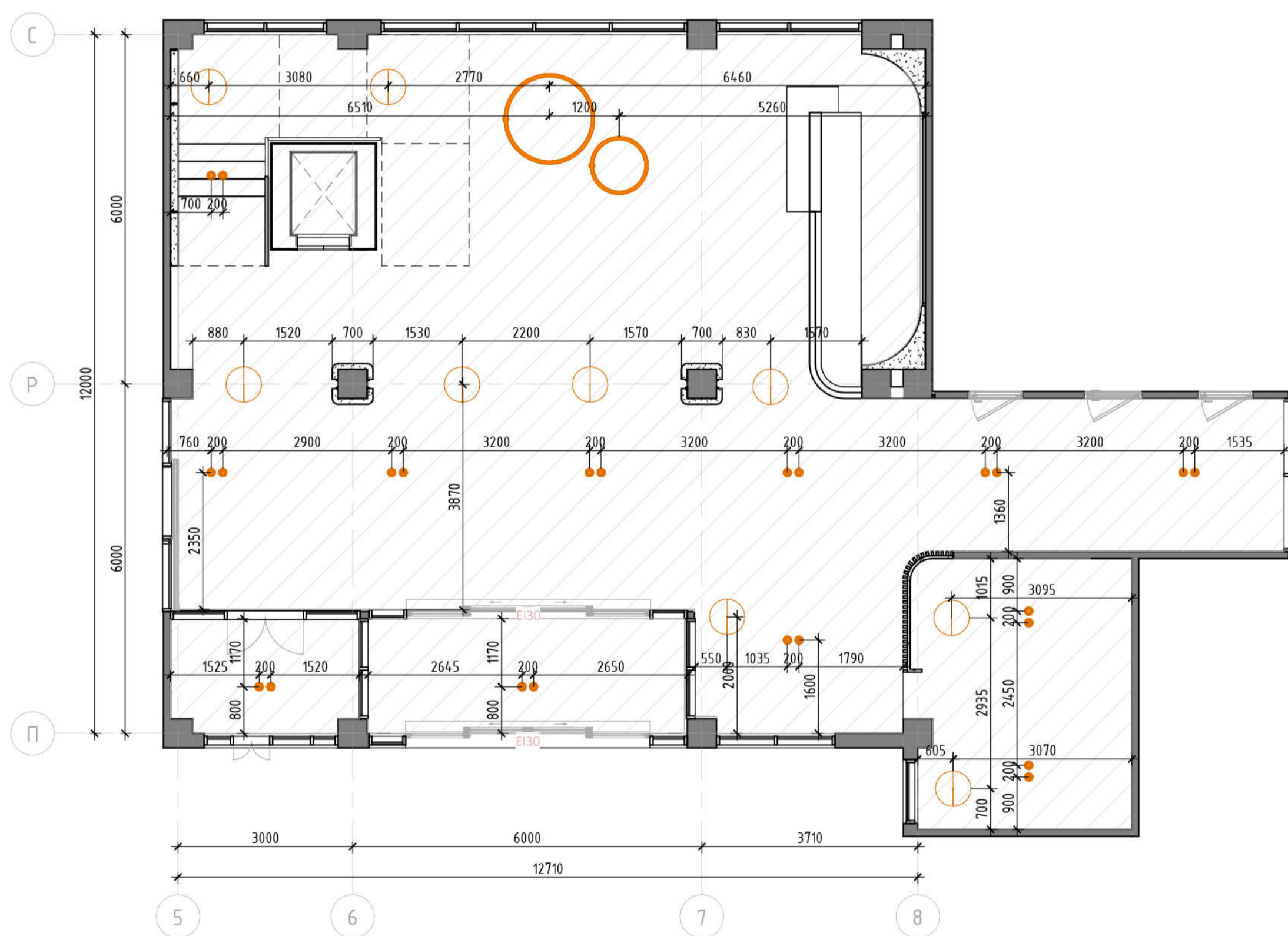
План стелі та розташування світильників М 1:50
