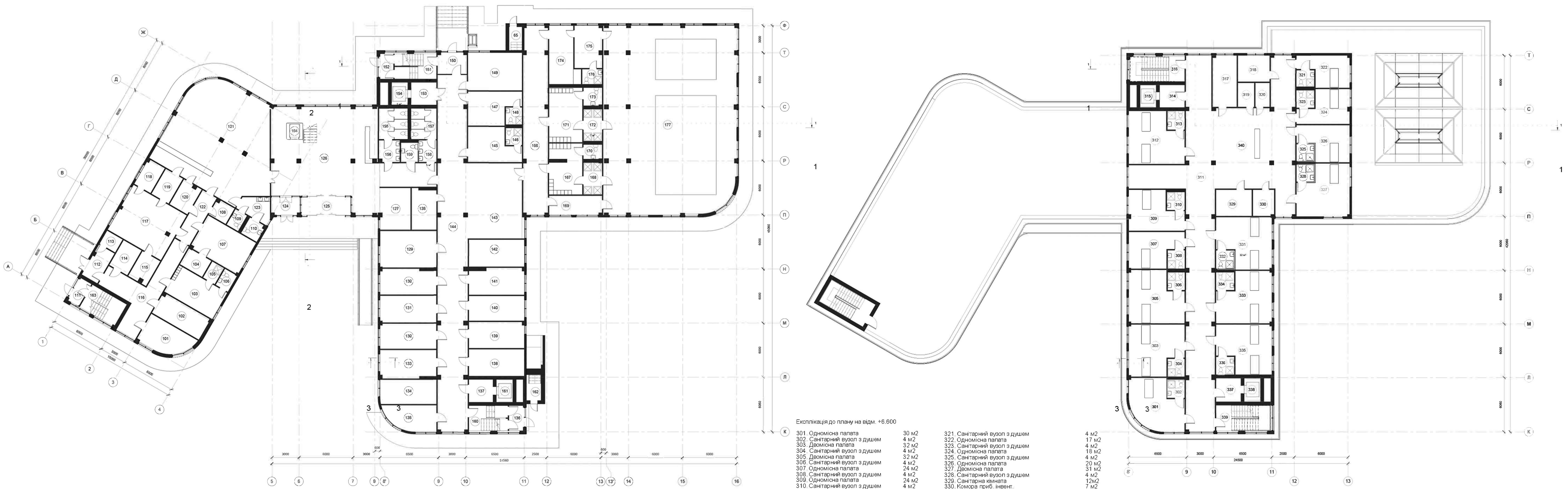
ПЛАН НА ВІДМІТЦІ +0.000 М 1:100
