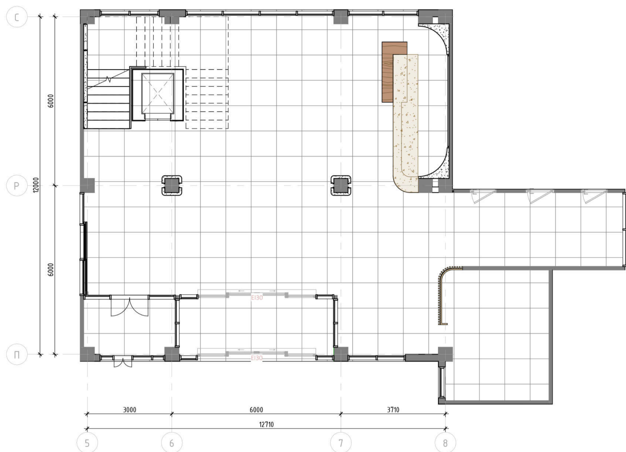
План підлоги та розташування меблів М 1:50
