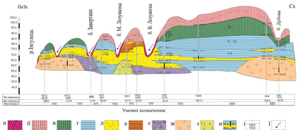
Рис. 2 – Геологічний розріз осадового чохла по лінії I-I (рис. 1) (за Є.І. Варьохом, з доповненнями); а – ґрунтово-рослинний шар; б – суглинки лесоподібні жовто-бурі, палеві з прошарками реліктових ґрунтів; в – суглинки червоно-бурі; г – глини сірі, зеленувато- та блакитно-сірі; д – піски; е – глини червоно-бурі; є – кора вивітрювання кристалічних порід докембрію; ж – жильні апліто-пегматоїдні граніти; з – плагіограніт-мігматити; и – свердловини; і – номери свердловин; ї – місця утворення техногенно-природного травертину
