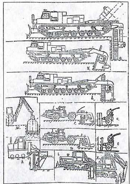
Схеми землерийних машин на українській ходовій базі (техніка НДІ БДІТ):
