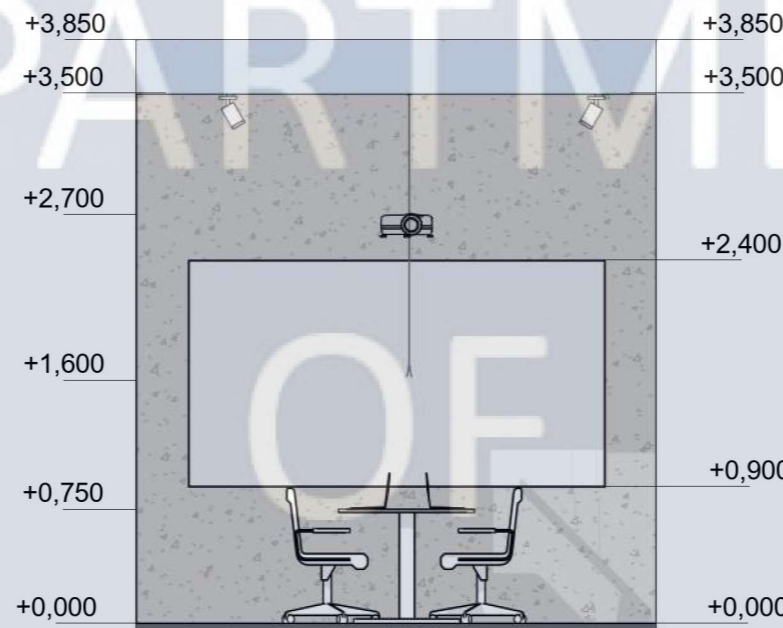
Розгортка 17 - 18 1 : 50
