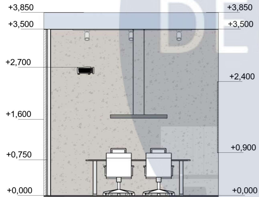
Розгортка 20 - 17 1 : 50
