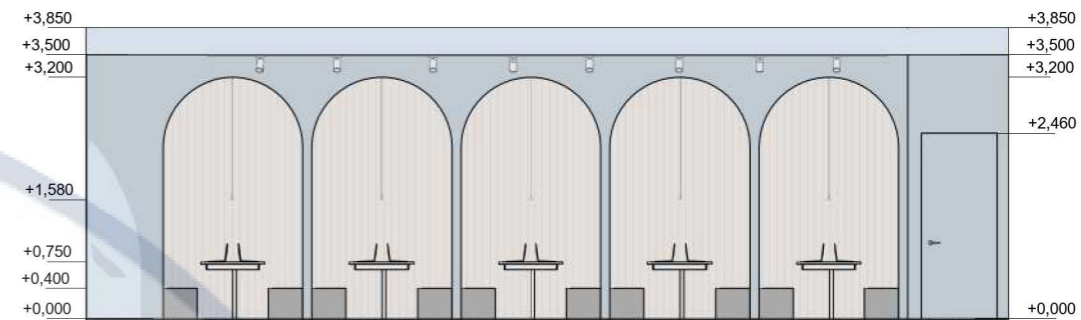
Розгортка 2 - 3 1 : 100
