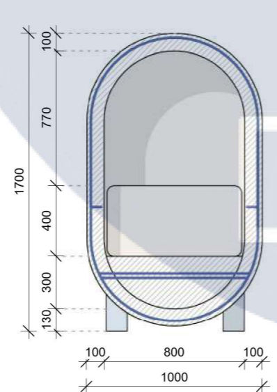
Поперечний переріз 1:30
