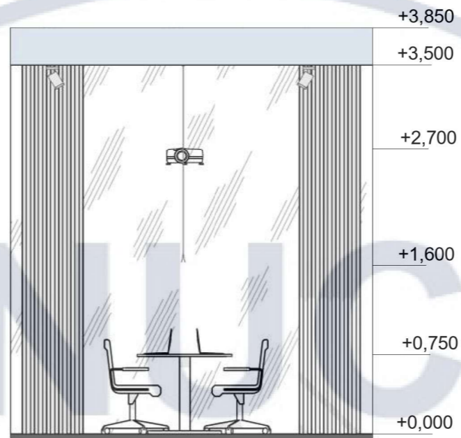
Розгортка 19 - 20 1 : 50
