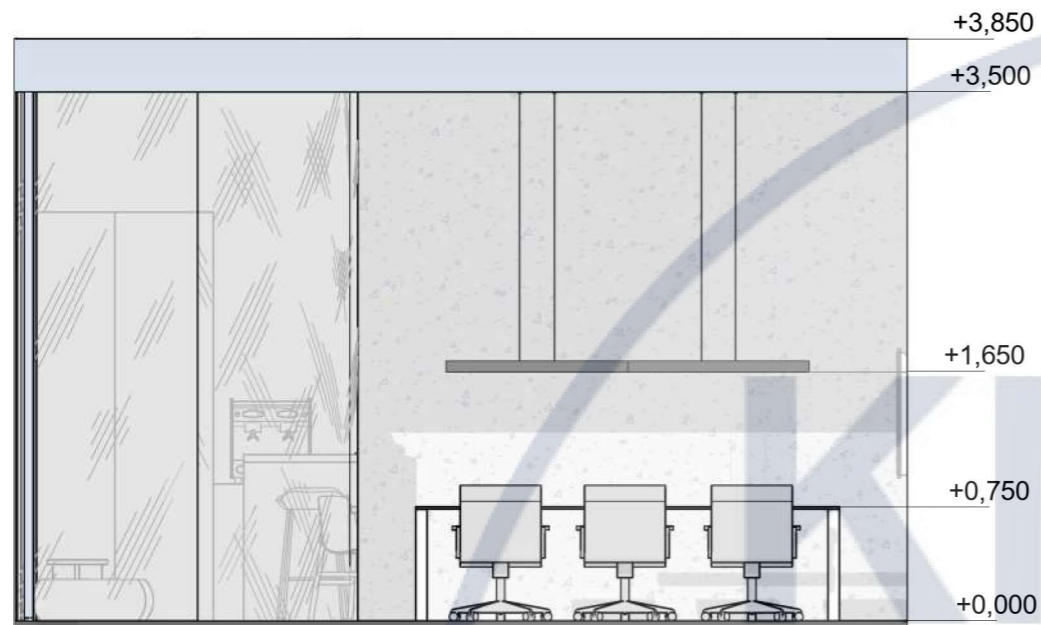
Розгортка 8 - 5 1 : 50
