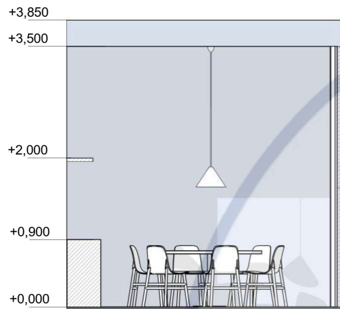
Розгортка 10 - 11 1 : 50
