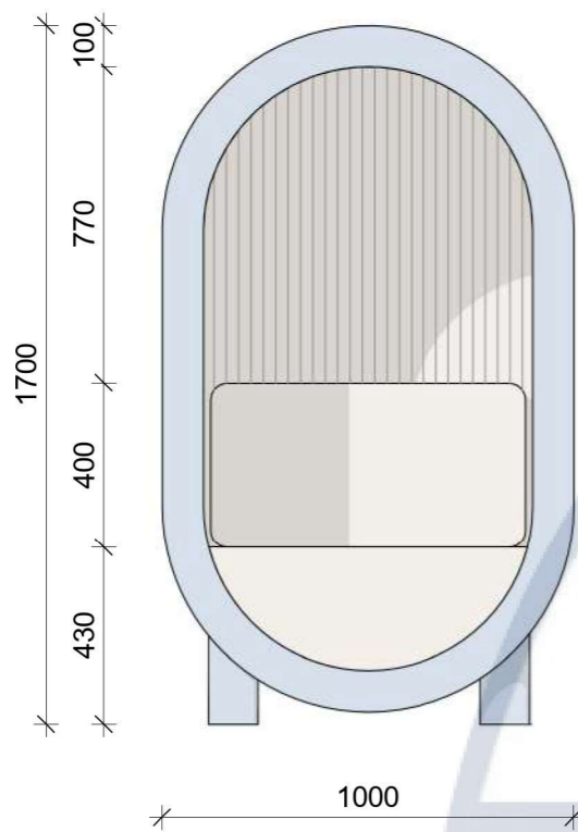
Вид спереду 1:20
