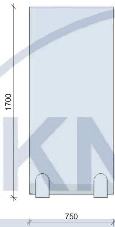
Вид збоку 1:20
