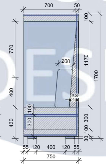
Повздовжний переріз 1:30
