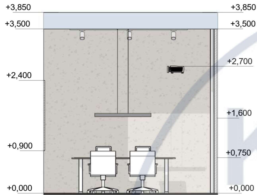
Розгортка 18 - 19 1 : 50
