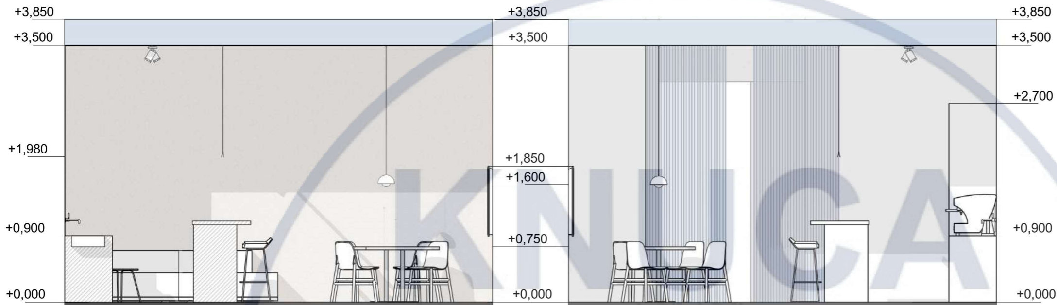
Розгортка 21 - 22 1 : 50
