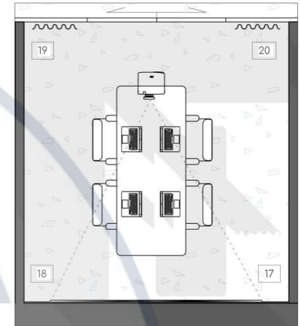
План меблів (маркування кімнати для демонстрацій) 1 : 50
