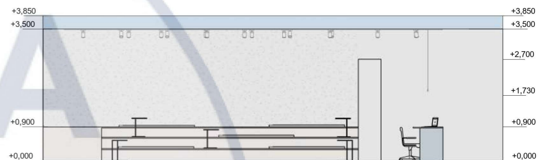
Розгортка 4 - 1 1 : 100
