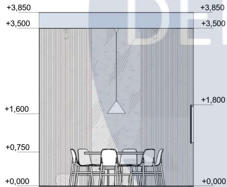
Розгортка 11 - 12 1 : 50
