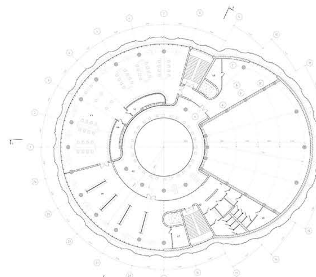
ПЛАН 3-ГО ПОВЕРХУ НА ВІДН. +11.700 М 1:100
