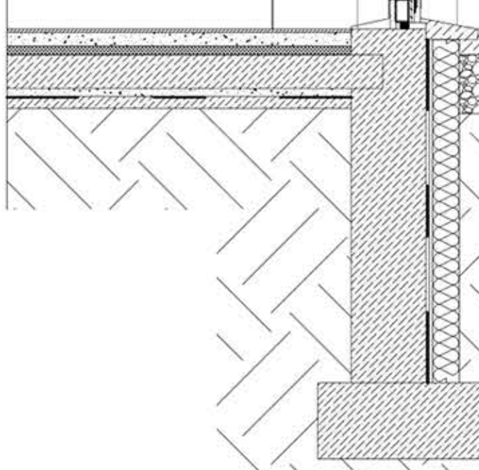
КОНСТРУКТИВНИЙ РОЗРІЗ ПО СТІНІ М 1:25
