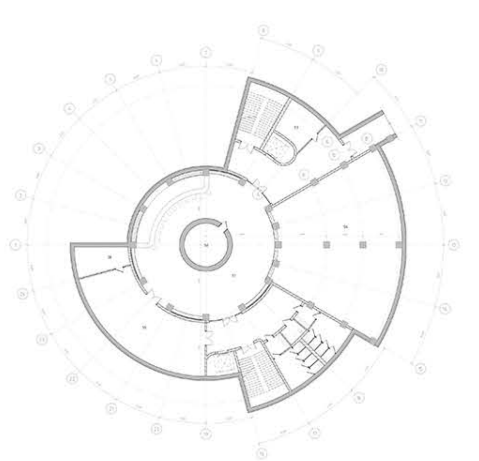
ПЛАН УКРИТТЯ НА ВІДМ. -3,600 М 1:100
