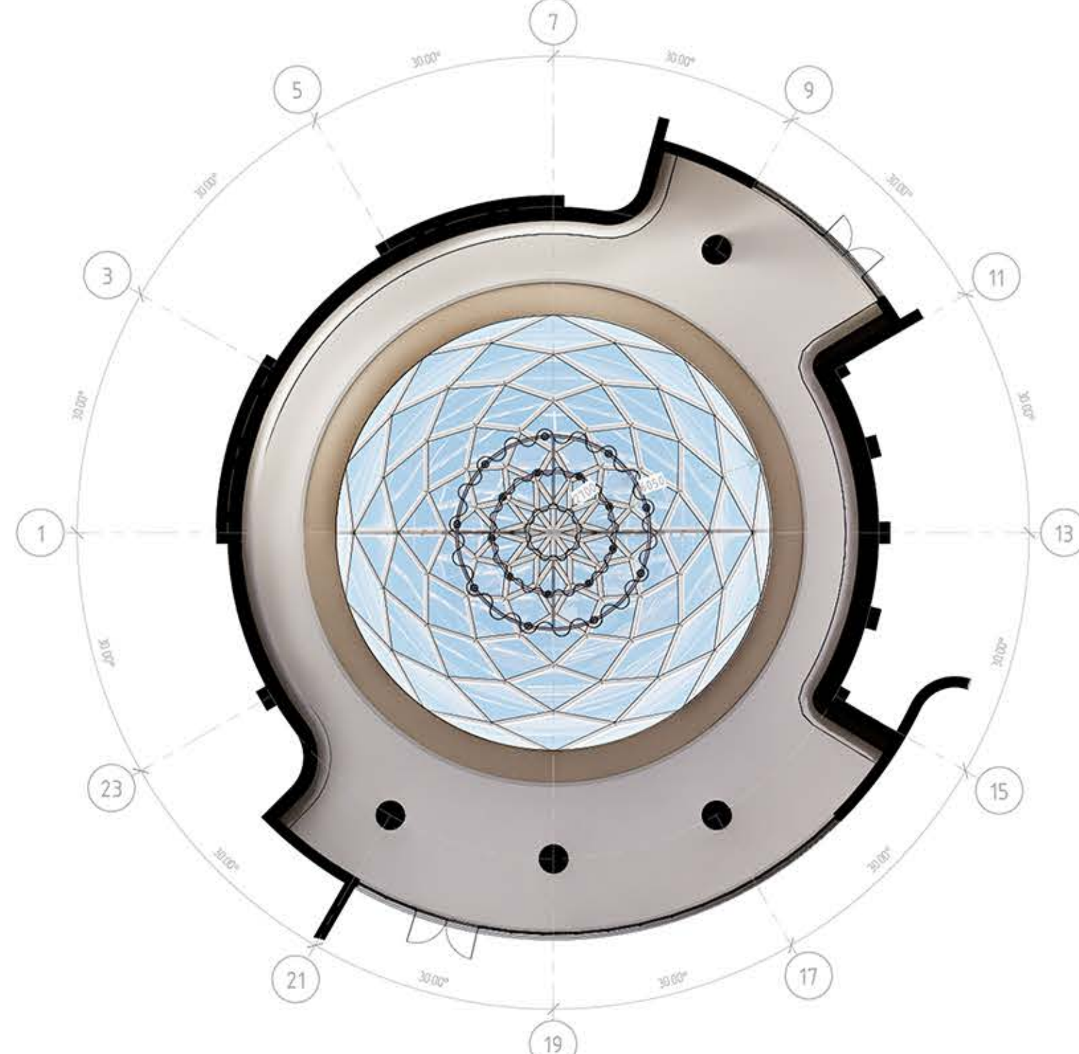
ПЛАН СТЕЛІ ЧИТАЛЬНОЇ ЗАЛИ М 1:100
