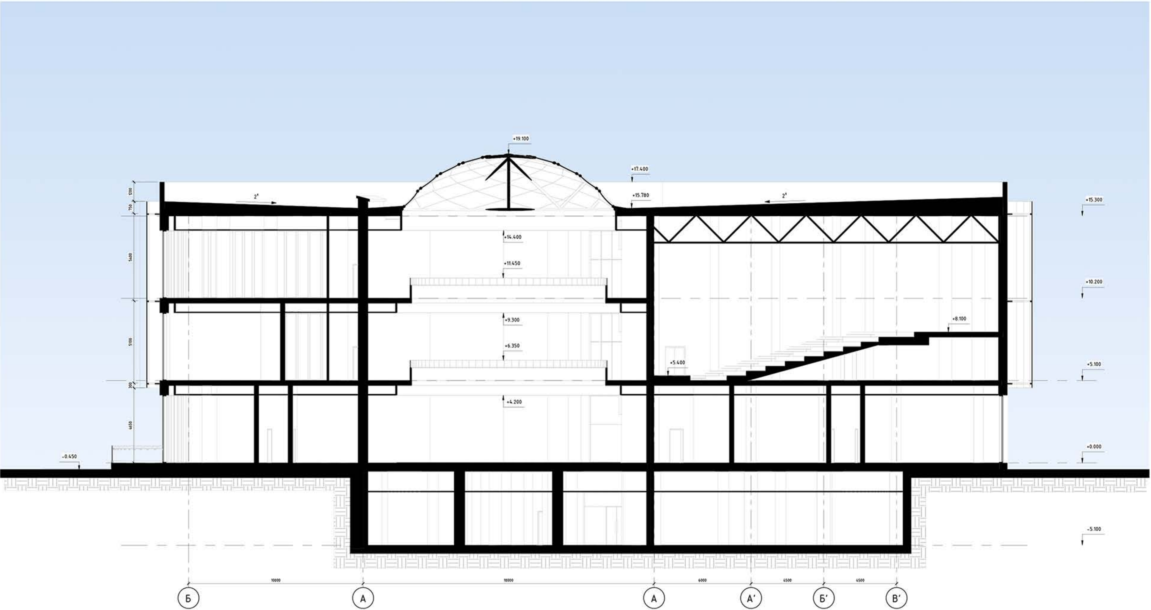
Р03РІ3 1-1 М 1:100
