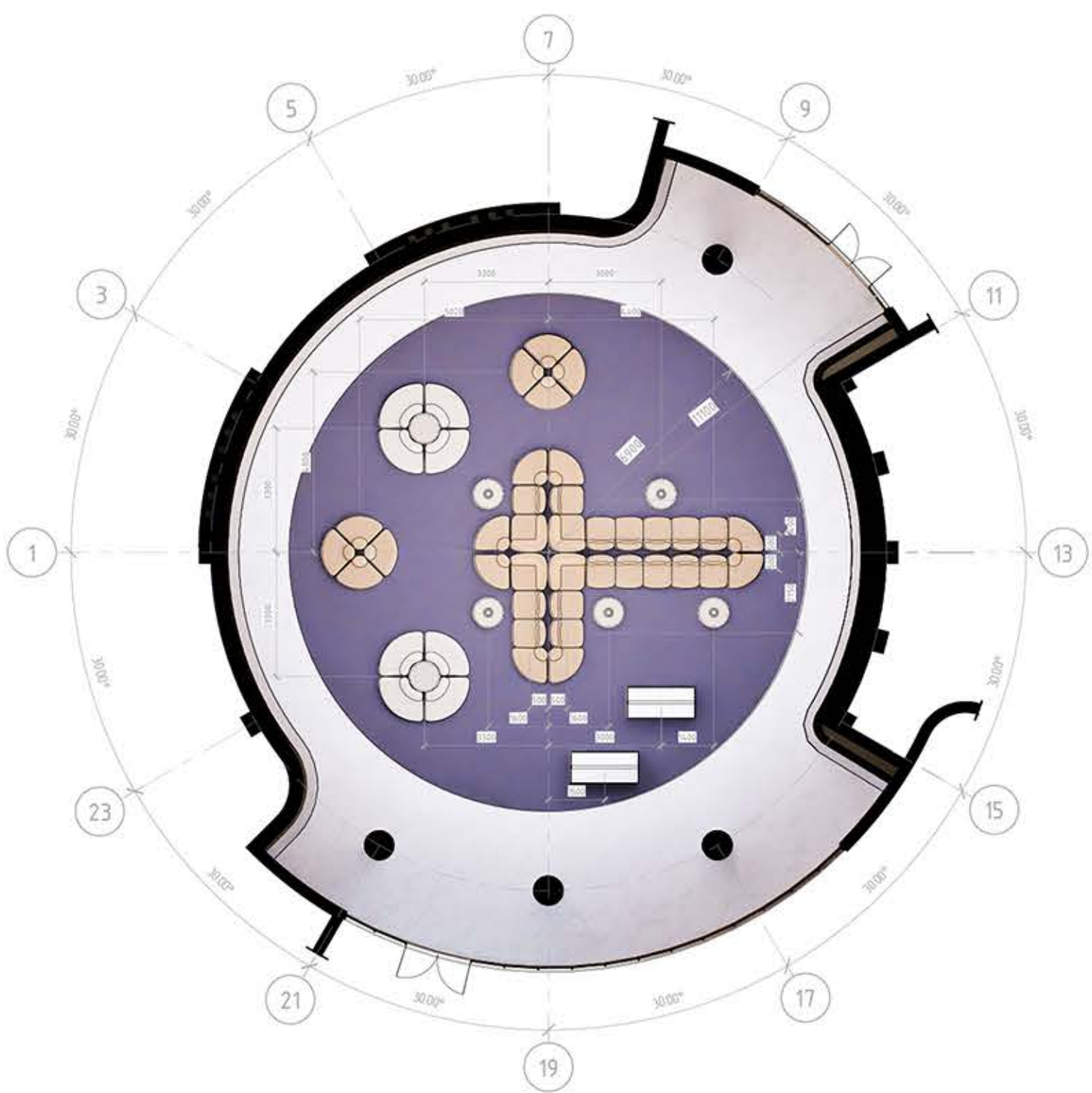
ПЛАН ПІДЛОГИ ЧИТАЛЬНОЇ ЗАЛИ М 1:100
