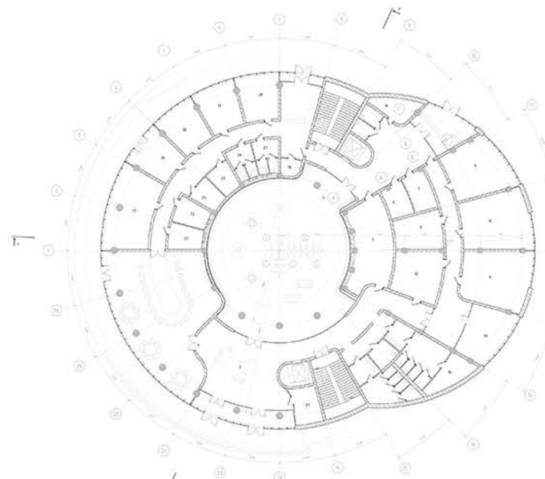
ПЛАН 1-ГО ПОВЕРХУ НА ВІДН. 1:500 М 1:100
