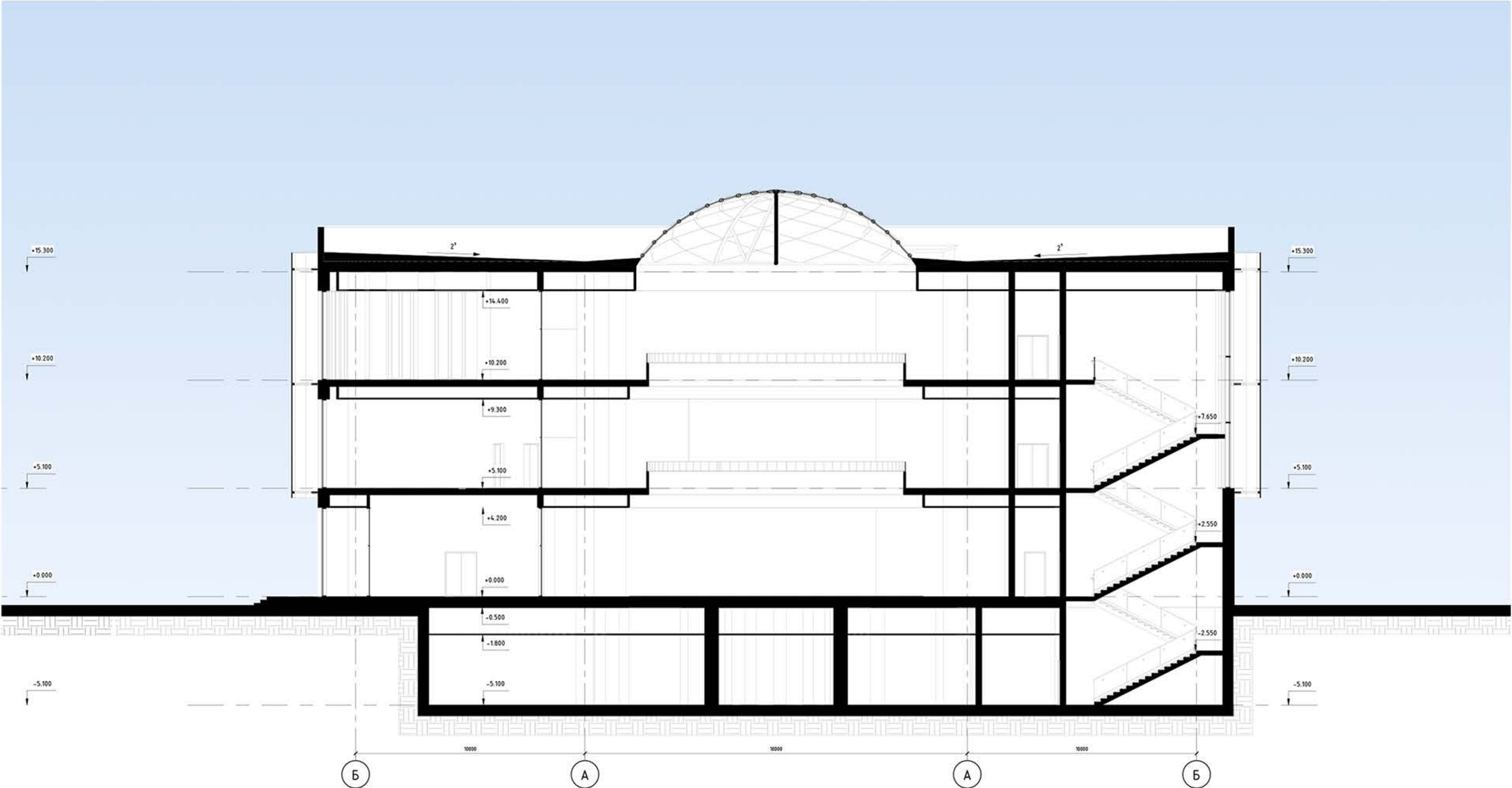
Р03РІ3 2-2 М 1:100
