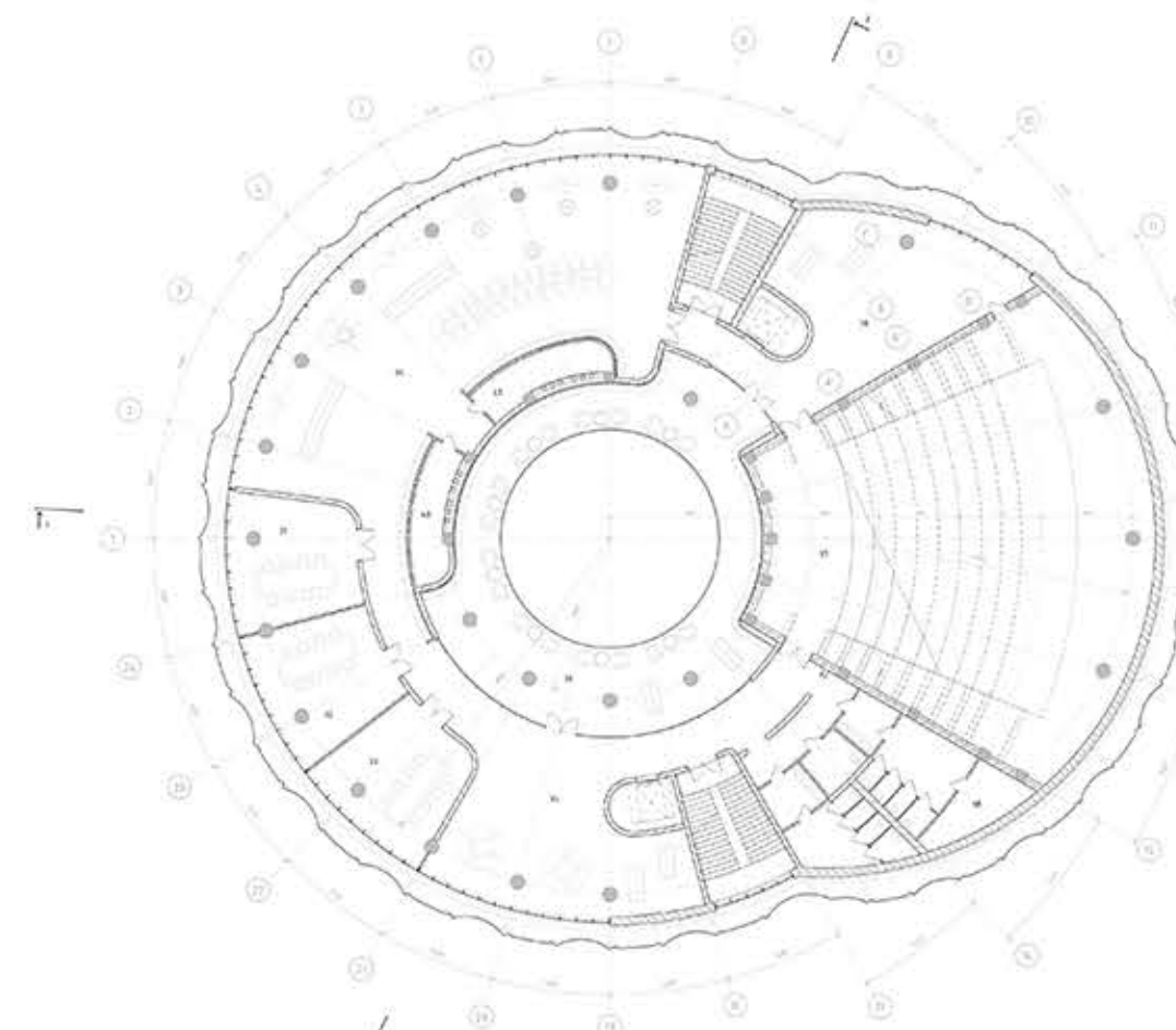
ПЛАН 2-ГО ПОВЕРХУ НА ВІДН. +6.600 М 1:100
