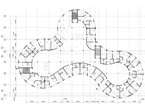
План поверху на відмітці +4.000 М 1:200
