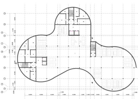
План поверху на відмітці -5.000 М 1:200
