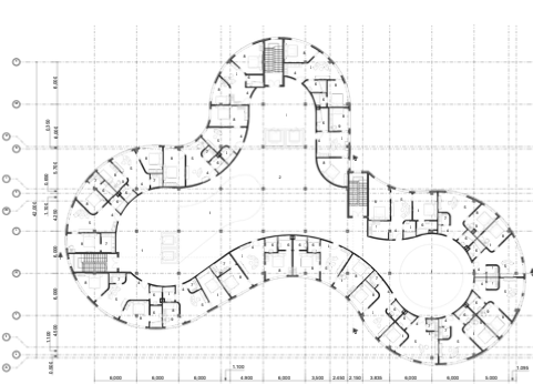
План поверху на відмітці +8.000 М 1:200
