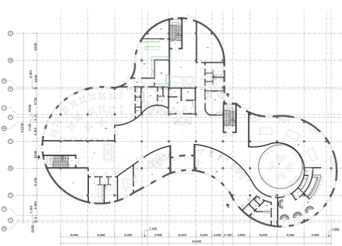
План поверху на відмітці 0.000 М 1:200
