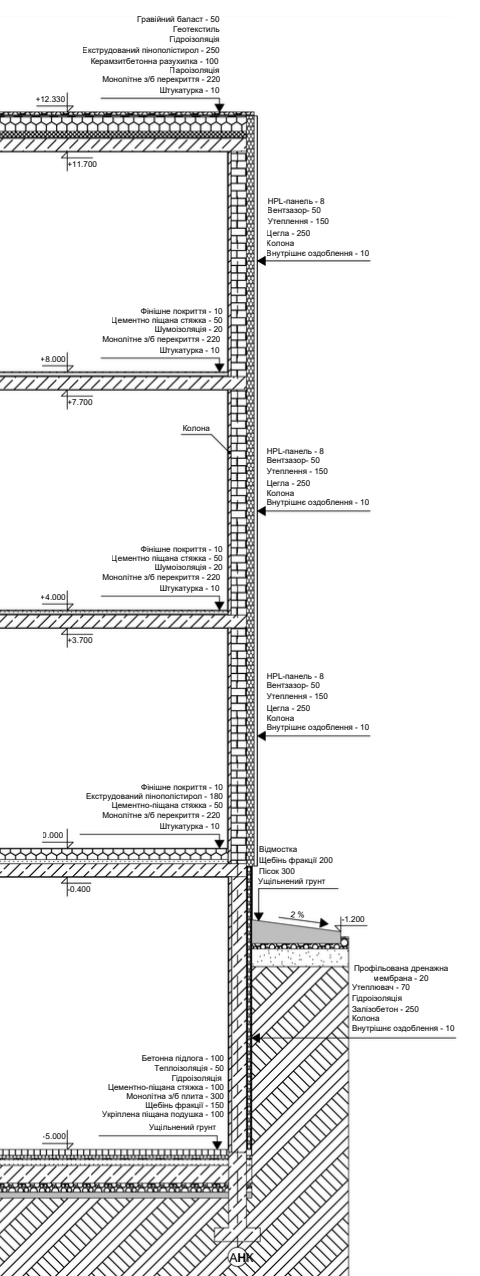
Розріз по зовнішній стіні М1:20
