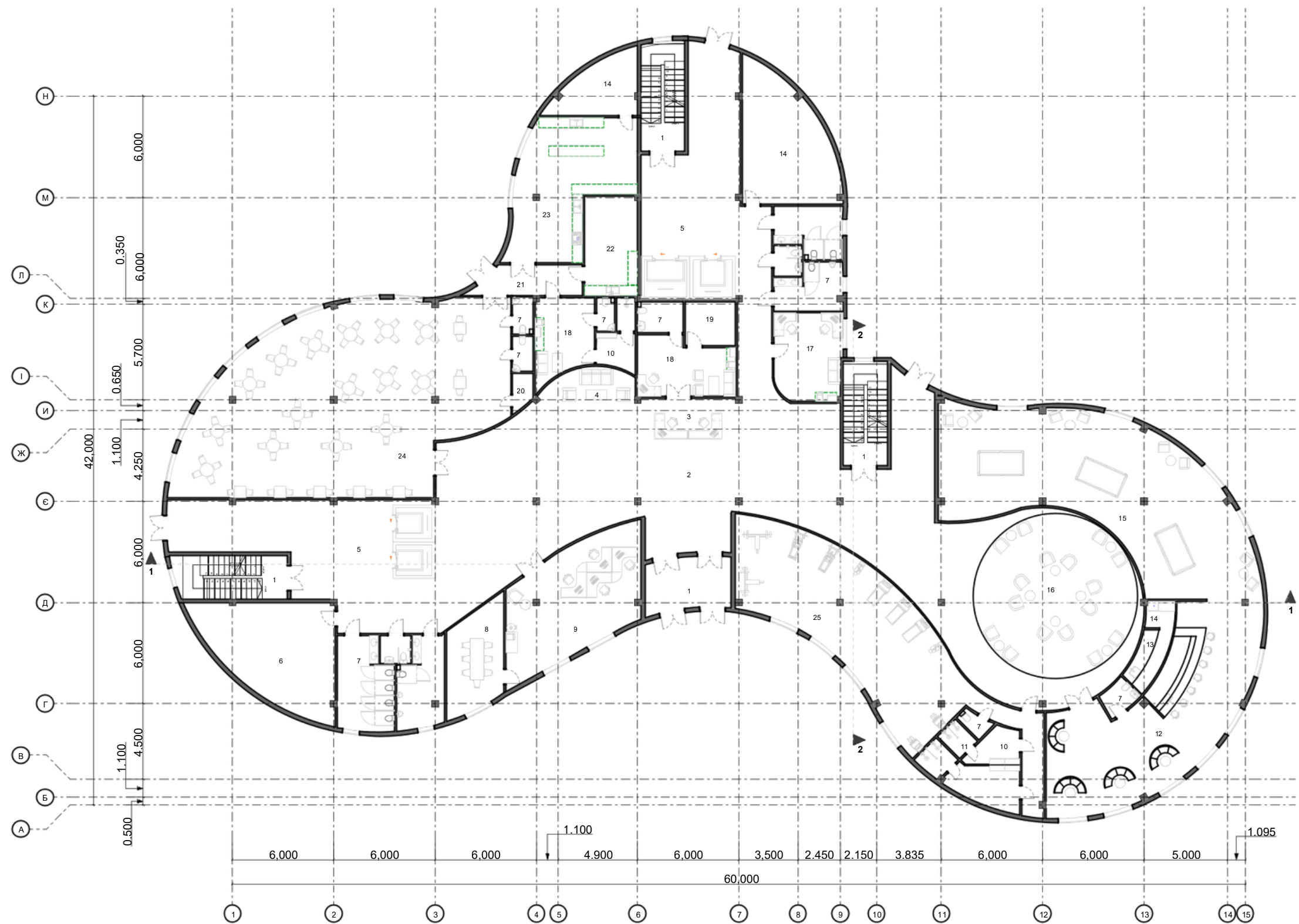
План поверху на відмітці 0.000 М 1:200
