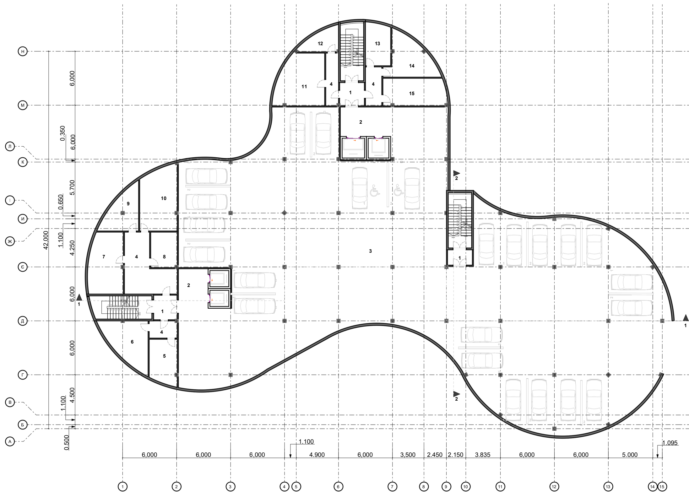
План поверху на відмітці -5.000 М 1:200
