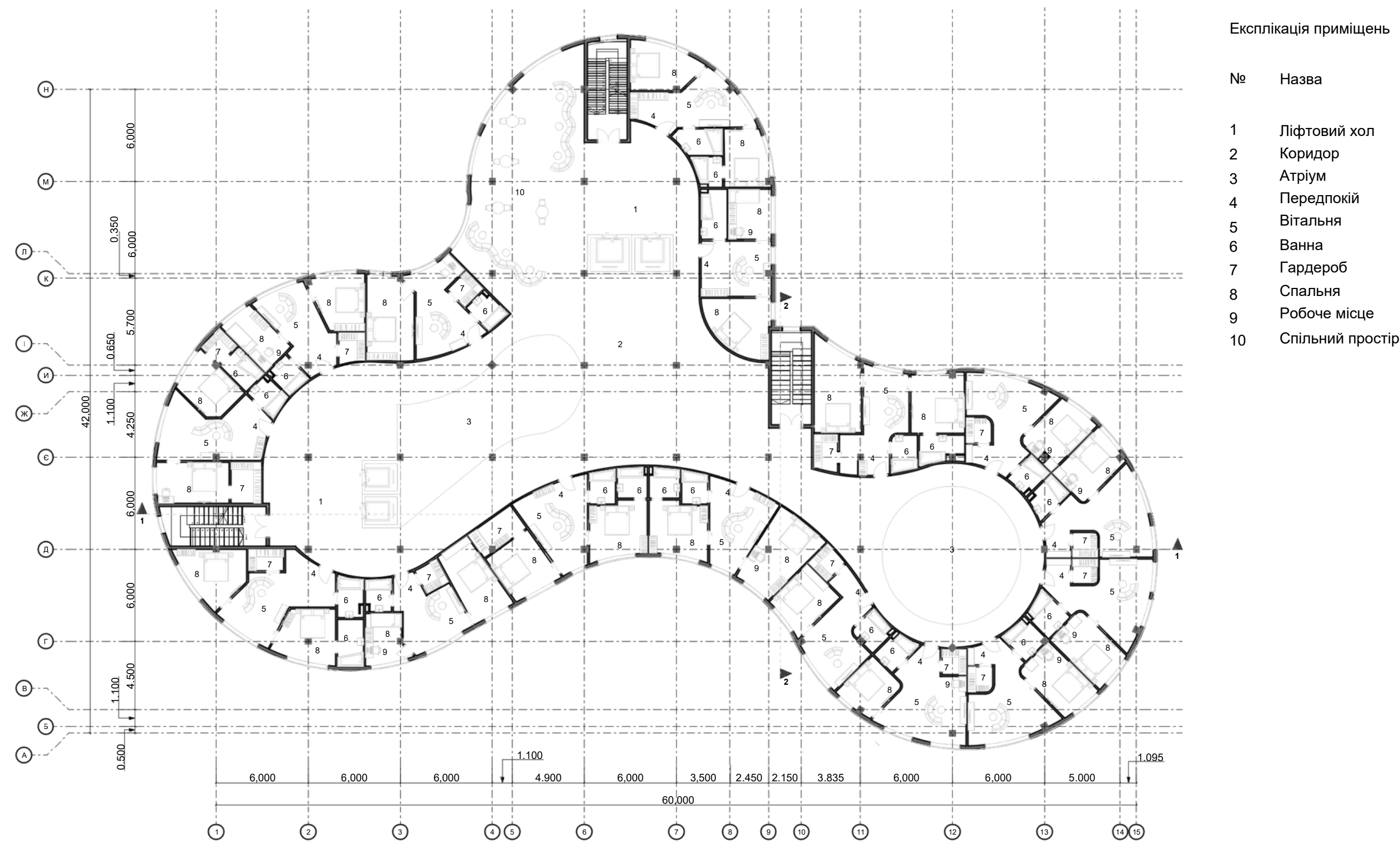
План поверху на відмітці +4.000 М 1:200
