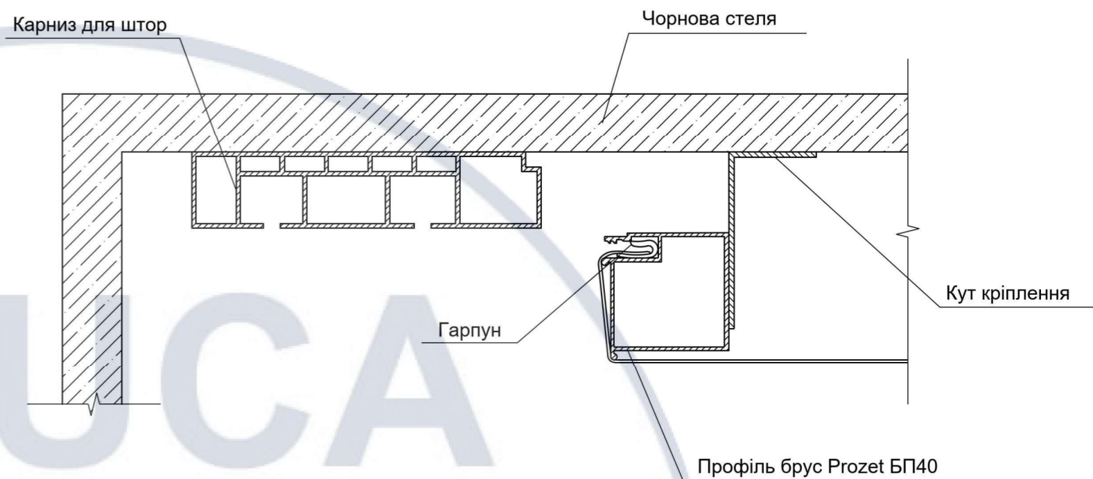
Вузол встановлення прихованого карнизу
