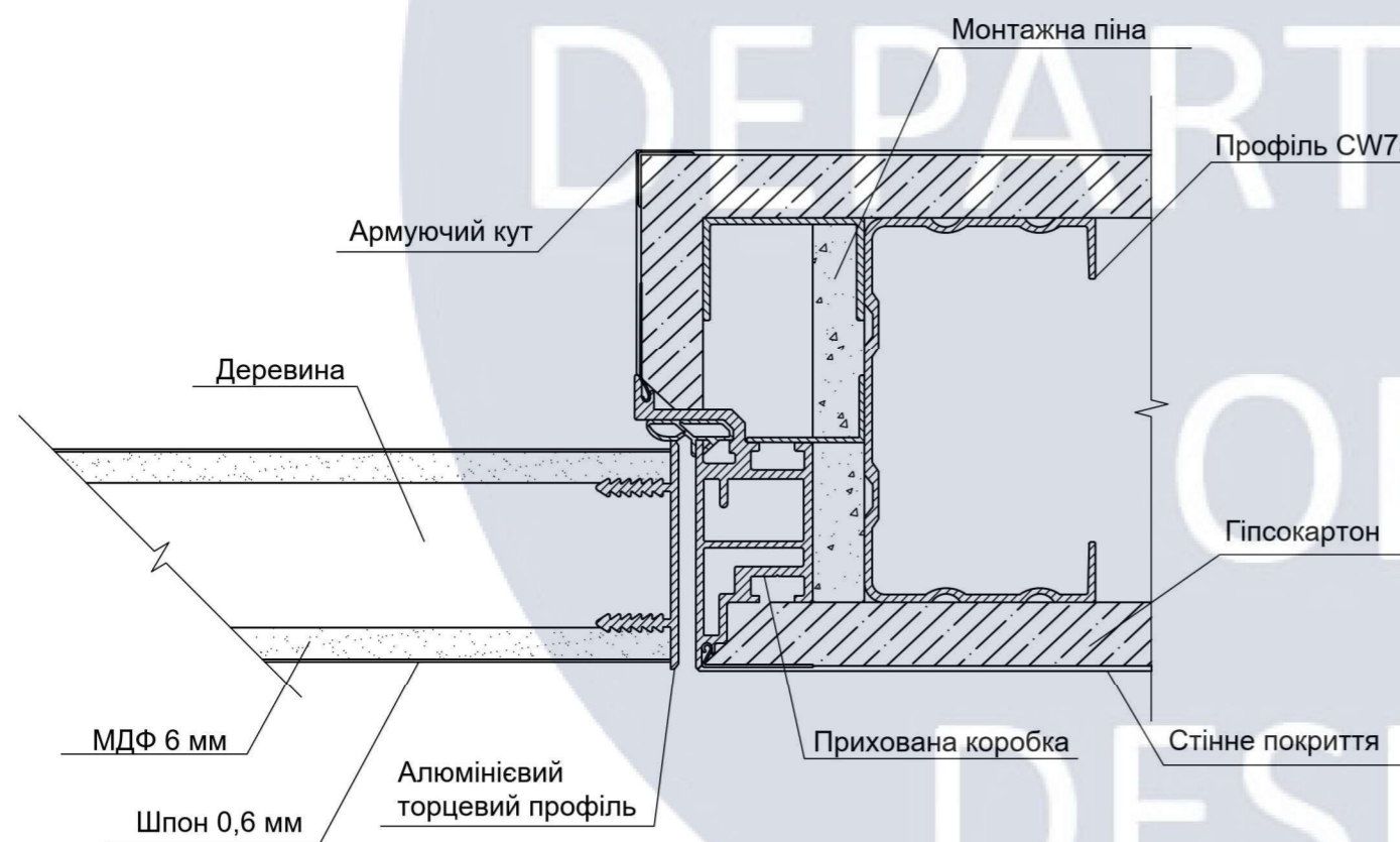
Вузол дверей прихованого монтажу
