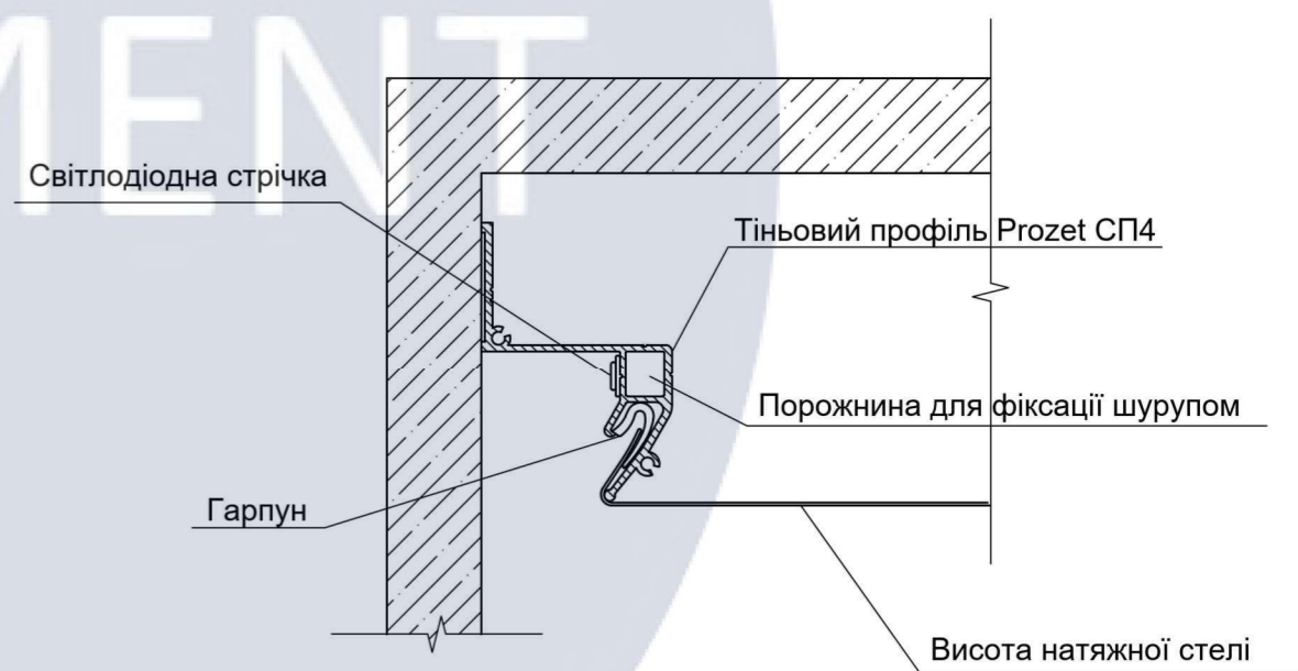
Вузол тіньового профілю
