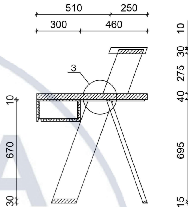
Розріз Б-Б
