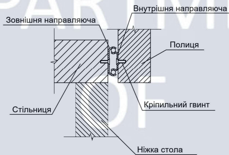
Вузол 1
