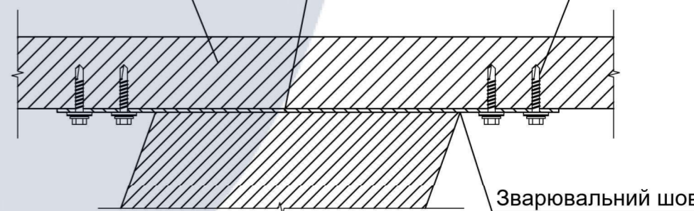
Металева пластина
