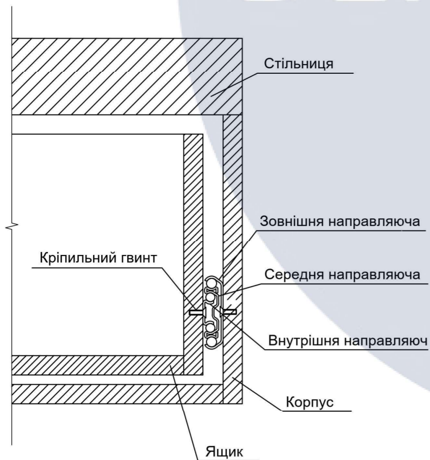
Вузол 2
