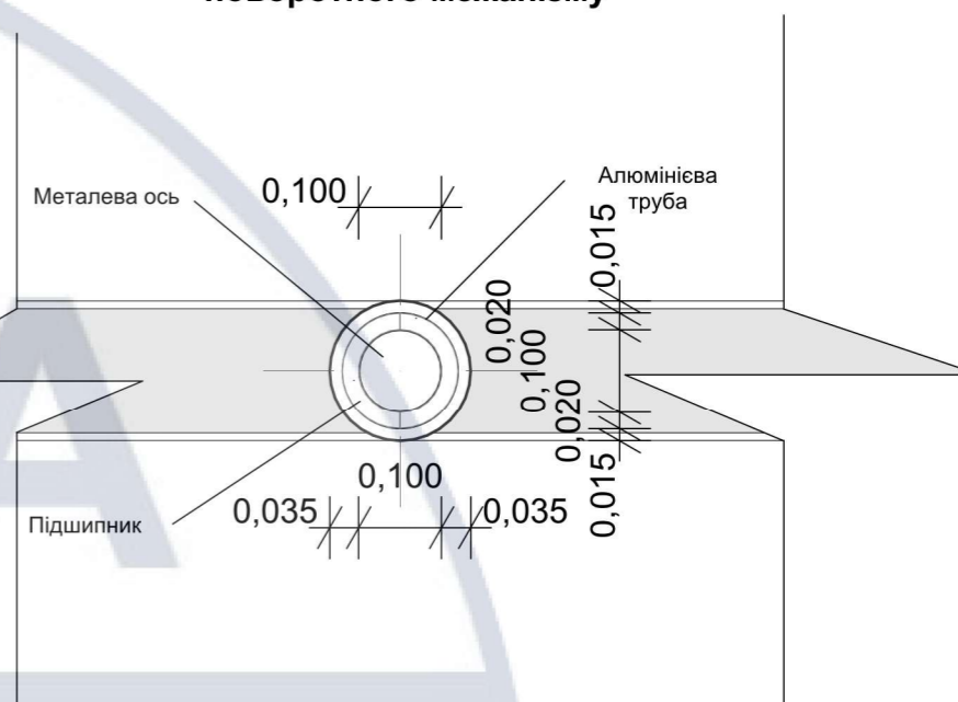
Вузол 1 Розміри підшипника поворотного механізму
