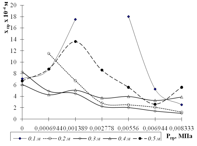
Рисунок 4. Залежність амплітуди коливань гравітаційного привантажувача від величини його тиску.
