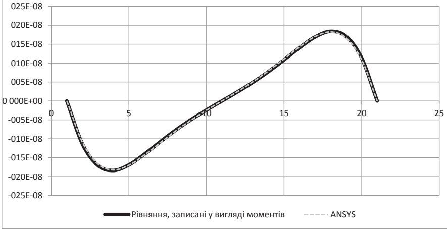
Графік №1 Горизонтальне переміщення точок 6-ї прямої, (м)
