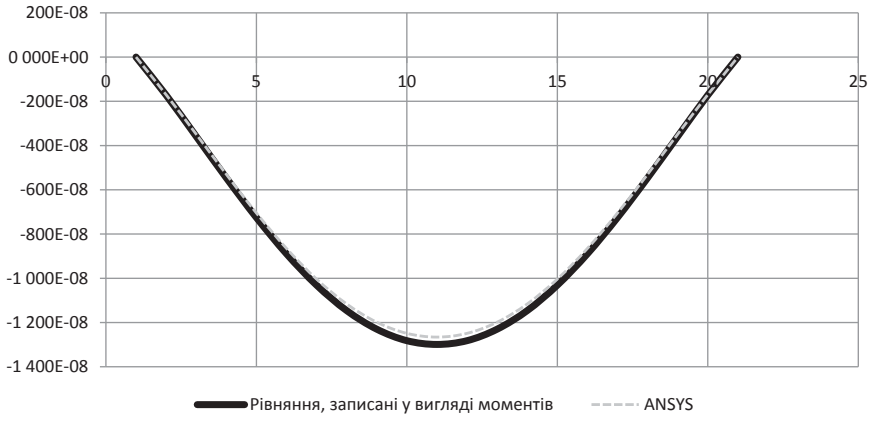
Графік №2 Вертикальне переміщення точок 6-ї прямої, (м)
