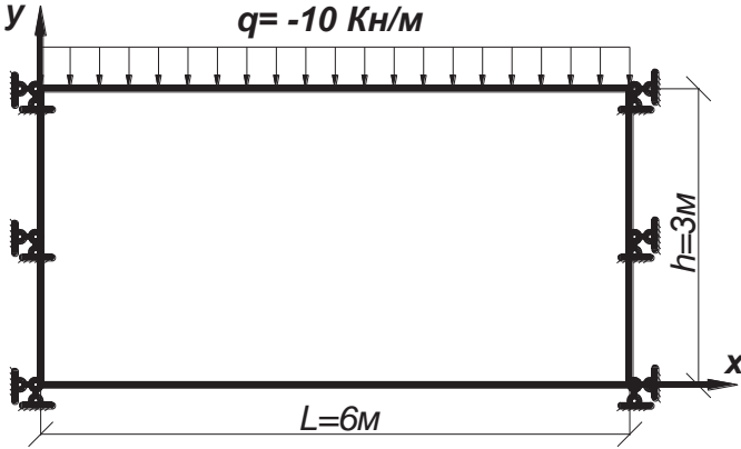
Рис.3. Дослідна модель балки-стінки.
