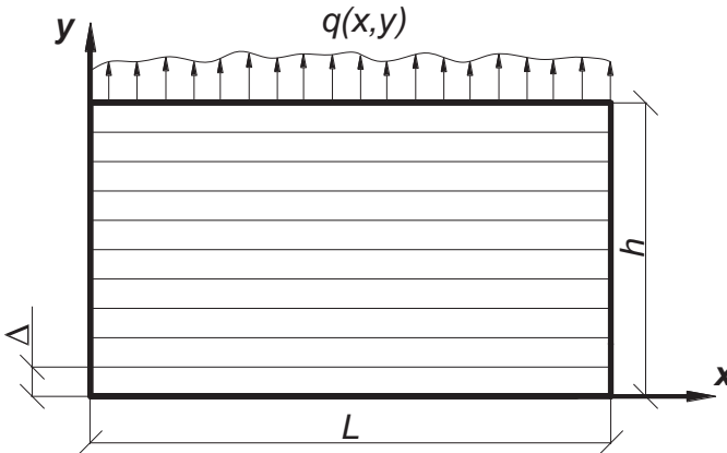
Рис.2. Плоский напружений стан балки-стінки.
