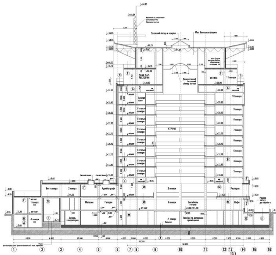
Рис. 12. Розріз
