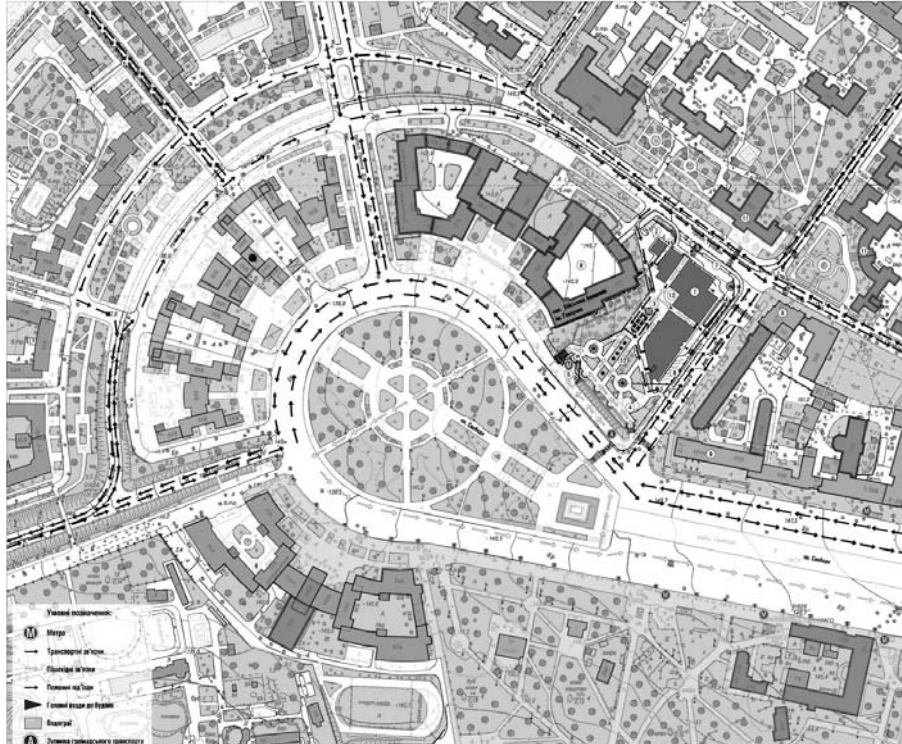
Рис. 4. Ситуаційний план. Транспортно - пішохідна схема
