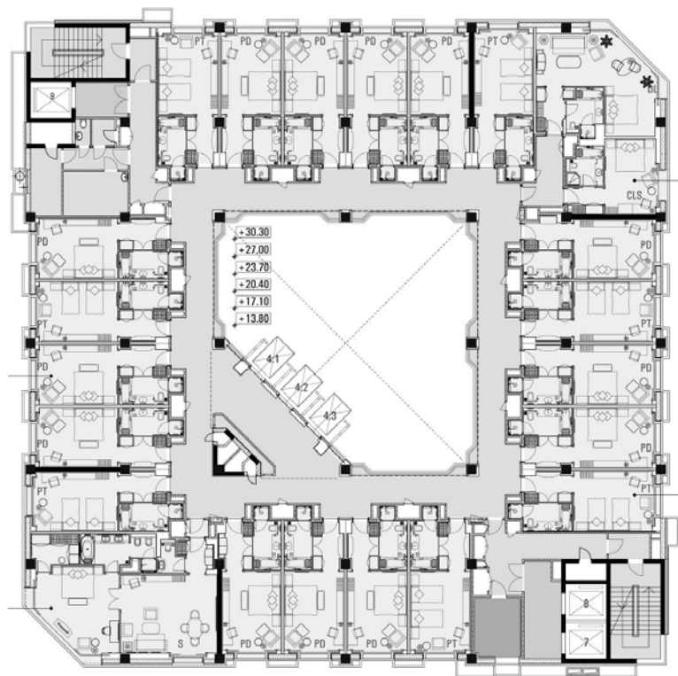
Рис. 11. План типового поверху
