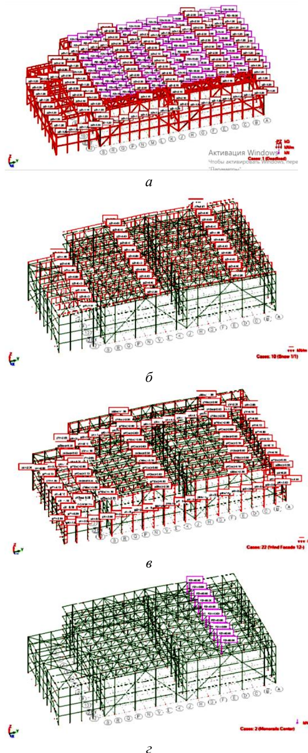
Рис. 3. Розрахункова схема в Robot Structure Analysis, завантажена навантаженнями: a – постійне; b – снігове; в – варіант вітрового навантаження; г – варіант кранового навантаження
