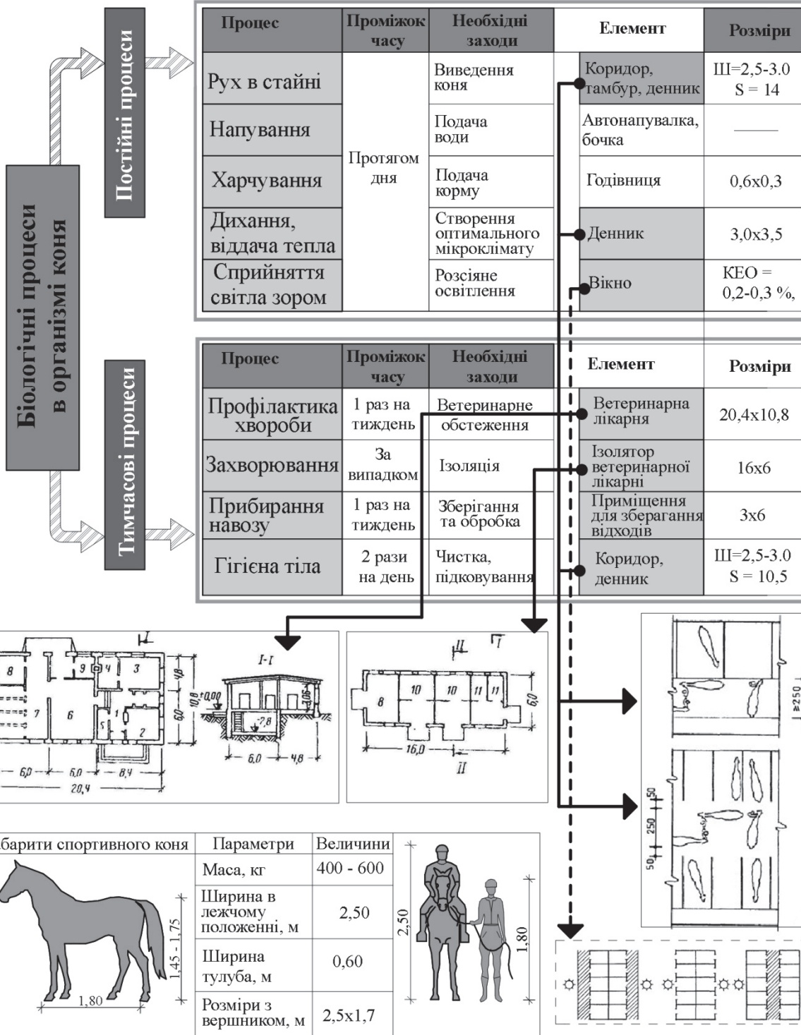
Рис. 3. Основні параметри приміщень стайні [1].
