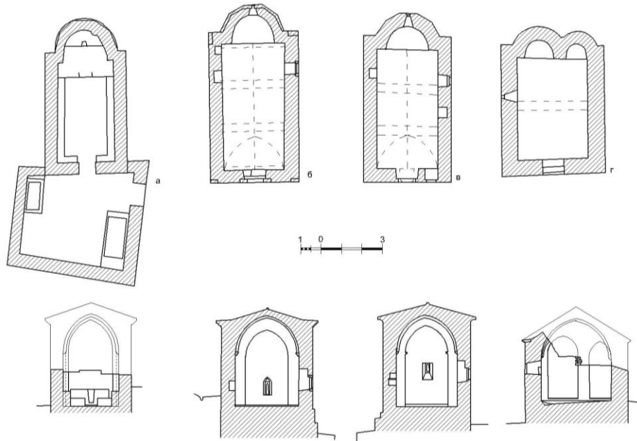
Іл.2. Плани та поперечні розрізи храмів.
